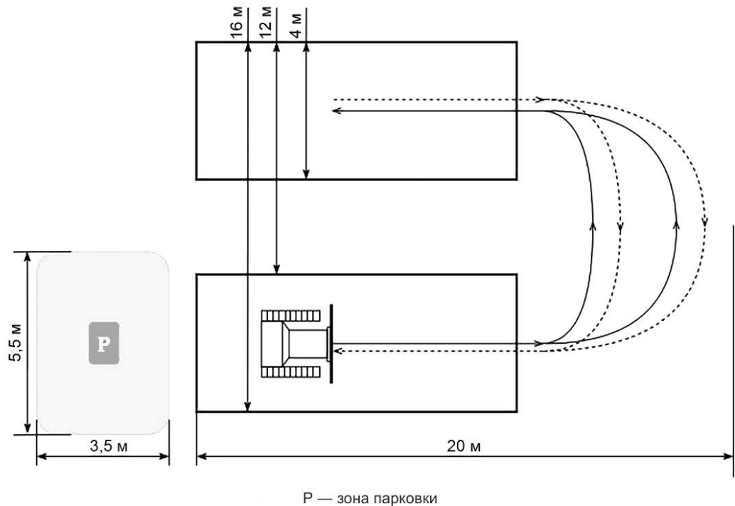
Рисунок А.1 — Минимальные размеры зоны движения ВАЗДСМ по криволинейной траектории (перемещение грунта)
