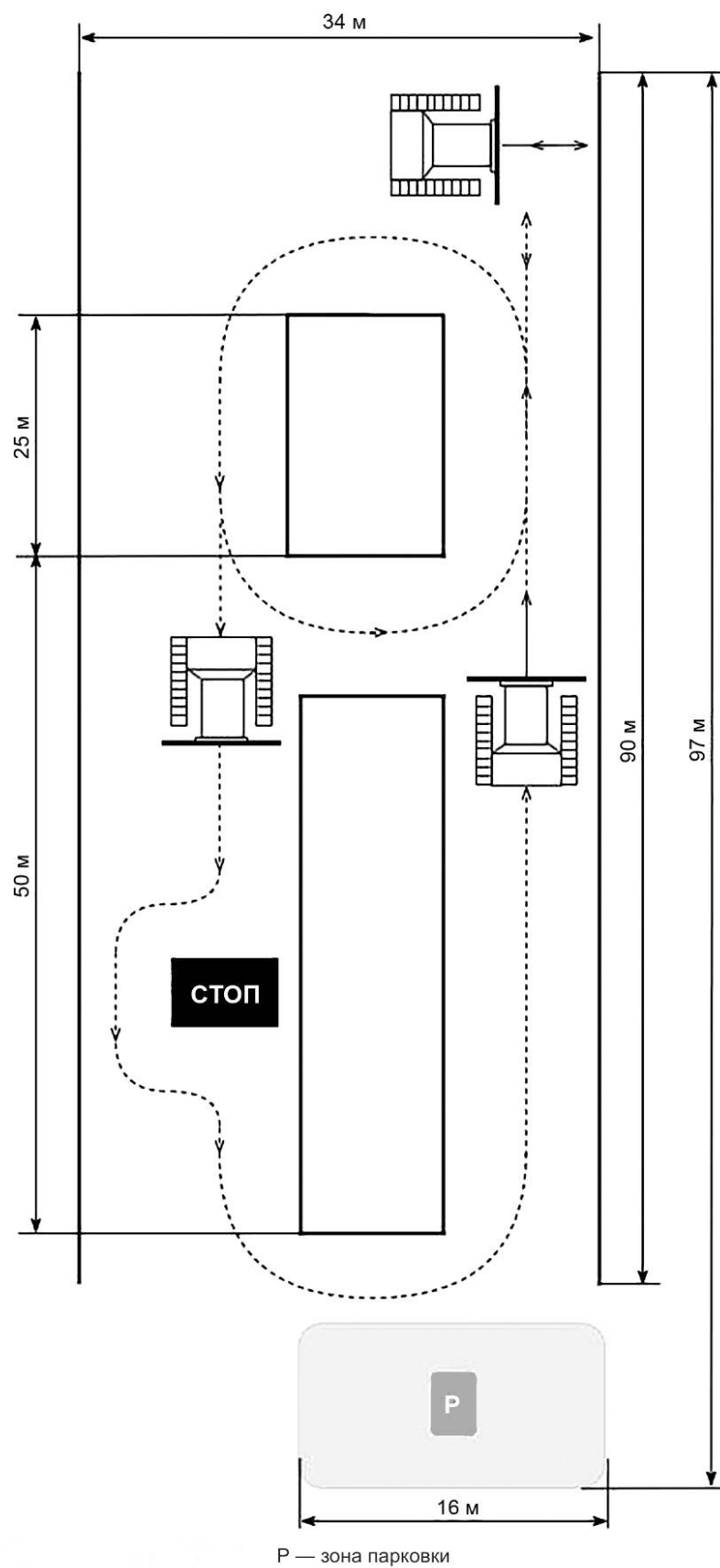
Рисунок А.3 — Минимальные размеры зоны управления в смешанном режиме (выемка грунта и расширение пространства выемки, перемещение грунта)
