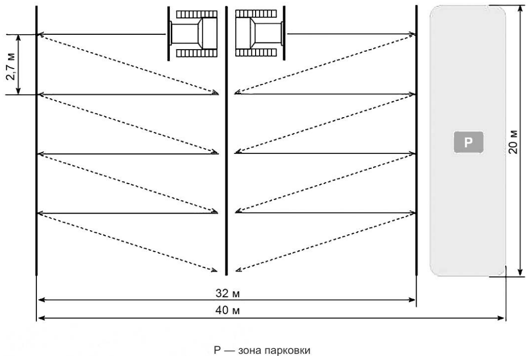
Рисунок А.2 — Минимальные размеры зоны группового движения (выемка грунта и расширение пространства выемки)
