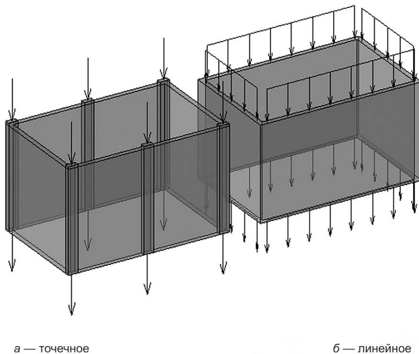
Рисунок 2 — Тип опирания модулей
