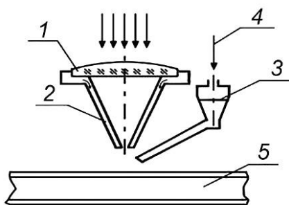
Рисунок В.1 — Схема устройства с коаксиальной подачей порошка
