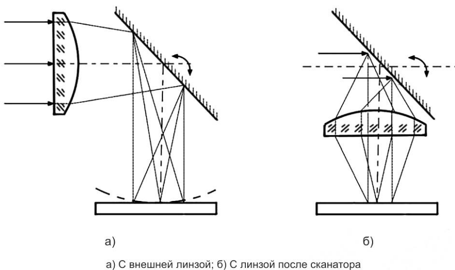
Рисунок 6 — Сканаторы с гальваническим зеркальным подвесом
