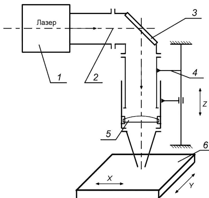
1 — лазер; 2 — лучепровод; 3 — поворотное зеркало; 4 — механизм перемещения по координате Z; 5 — фокусирующая линза; 6 — стол с перемещениями по координатам X—Y
