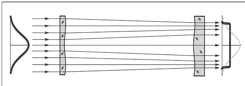
Рисунок 3 — Схема преобразования гауссового пучка в пучок равномерной интенсивности
