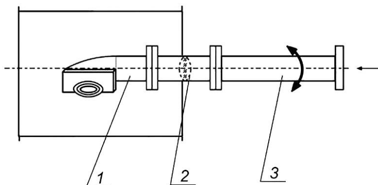
1 — поворотная ТГ с отклоняющим зеркалом, соплом и защитным стеклом; 2 — линза; 3 — штанга-удлинитель
