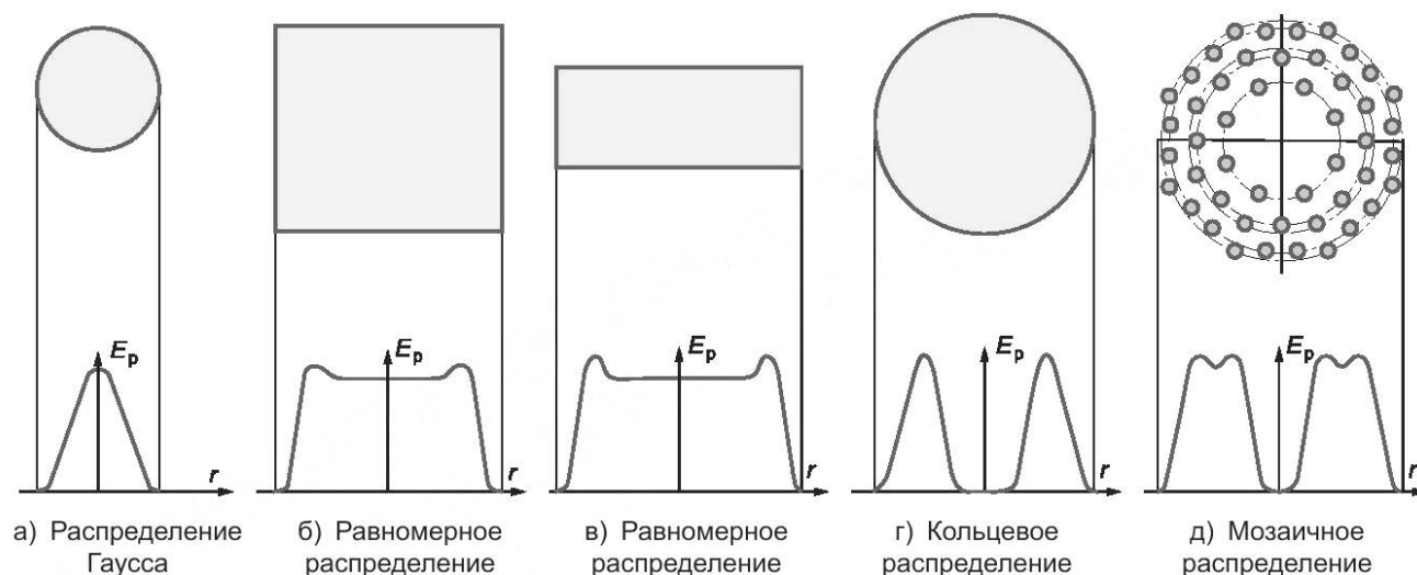
Рисунок 4 — Распределение плотности мощности лазерного излучения E_p
