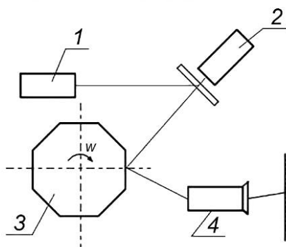
1 — лазер; 2 — система колеблющихся зеркал; 3 — полигональный зеркальный цилиндр; 4 — фокусатор
