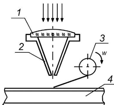
Рисунок В.2 — Схема устройства с боковой подачей порошка
