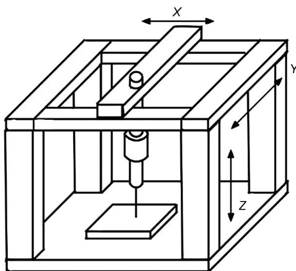
Рисунок 2 — Зеркальный лучепровод портального типа
