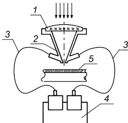
1 — линза; 2 — сопло; 3 — каналы для подачи порошков; 4 — двухкамерный питатель с подогревом и независимой подачей порошков; 5 — деталь
