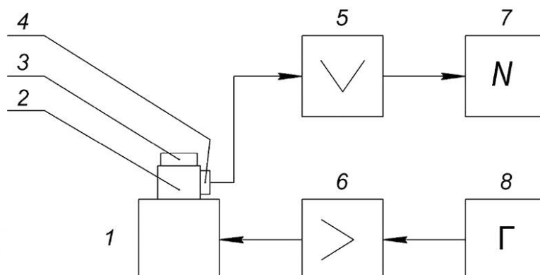
Рисунок 1 — Структурная схема обнаружения ПСПЧ методом регистрации акустических волн
