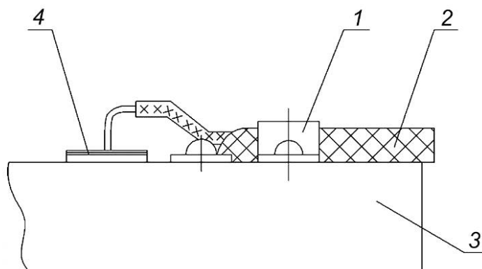
Рисунок А.2 — Конструкция пьезоэлектрического преобразователя
