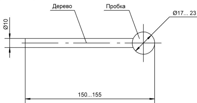
а) Молоточек с шарообразным бойком
