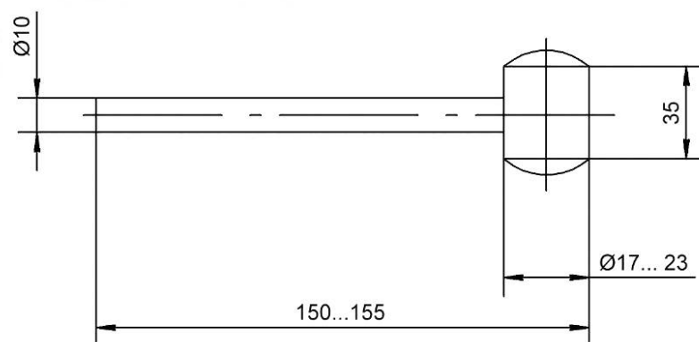
б) Молоточек с цилиндрическим бойком
