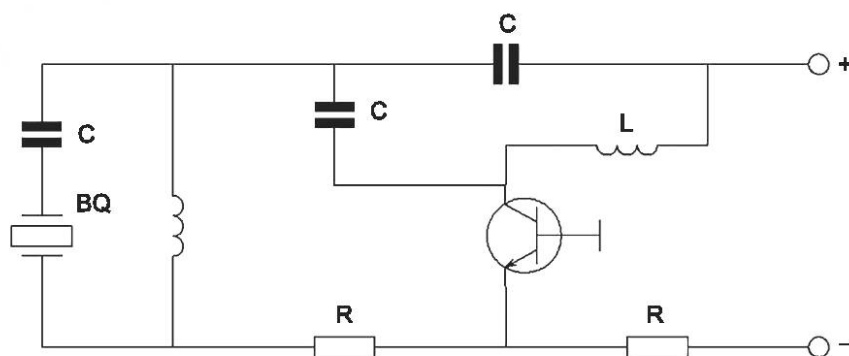
Рисунок В.4 — Генератор по схеме Колпитца до 300 МГц (резонатор в цепи обратной связи)
