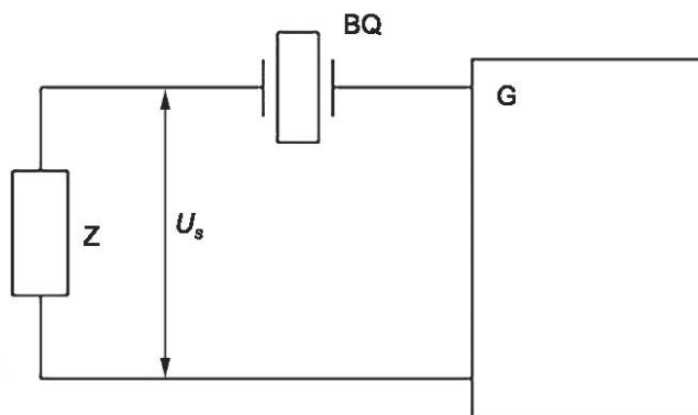
BQ — резонатор; Z — элемент, включенный последовательно с резонатором; G — схема применения резонатора; U_s — напряжение, измеренное на элементе, включенном последовательно к резонатору
