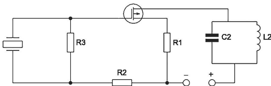
Рисунок В.3 — Генератор по схеме Пирса до 150 КГц (емкостная трехточка)
