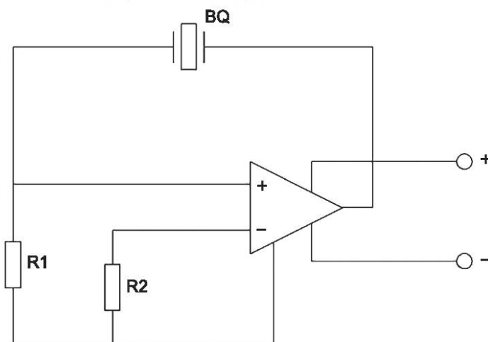
Рисунок В.2 — Низкочастотный генератор до 1 МГц
