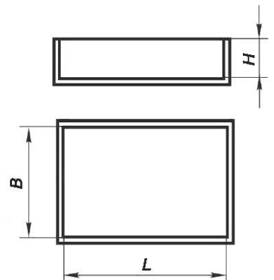
L — длина; B — глубина; H — высота Рисунок 4
