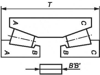
Конструктивное исполнение 09
