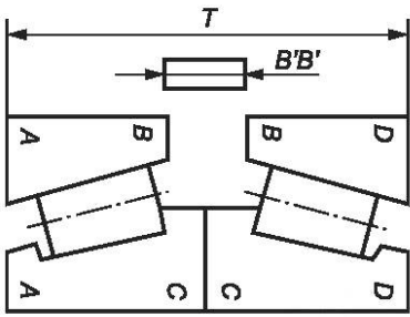
Конструктивное исполнение 52
