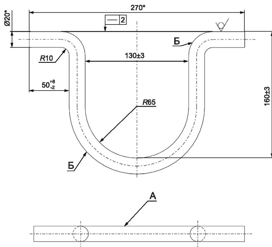
а) Исполнение -01
