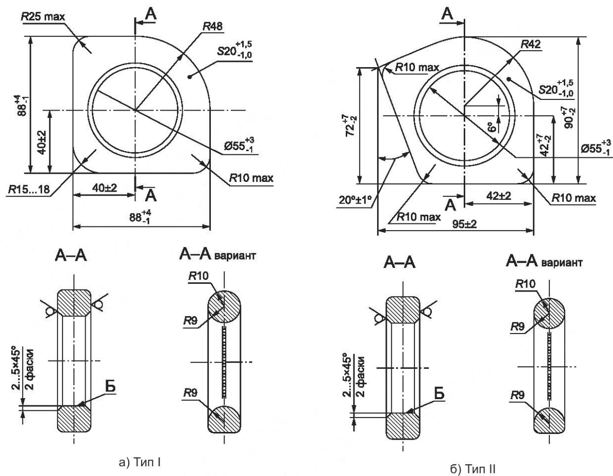
Рисунок 14 — Увязочные кольца типов I и II
