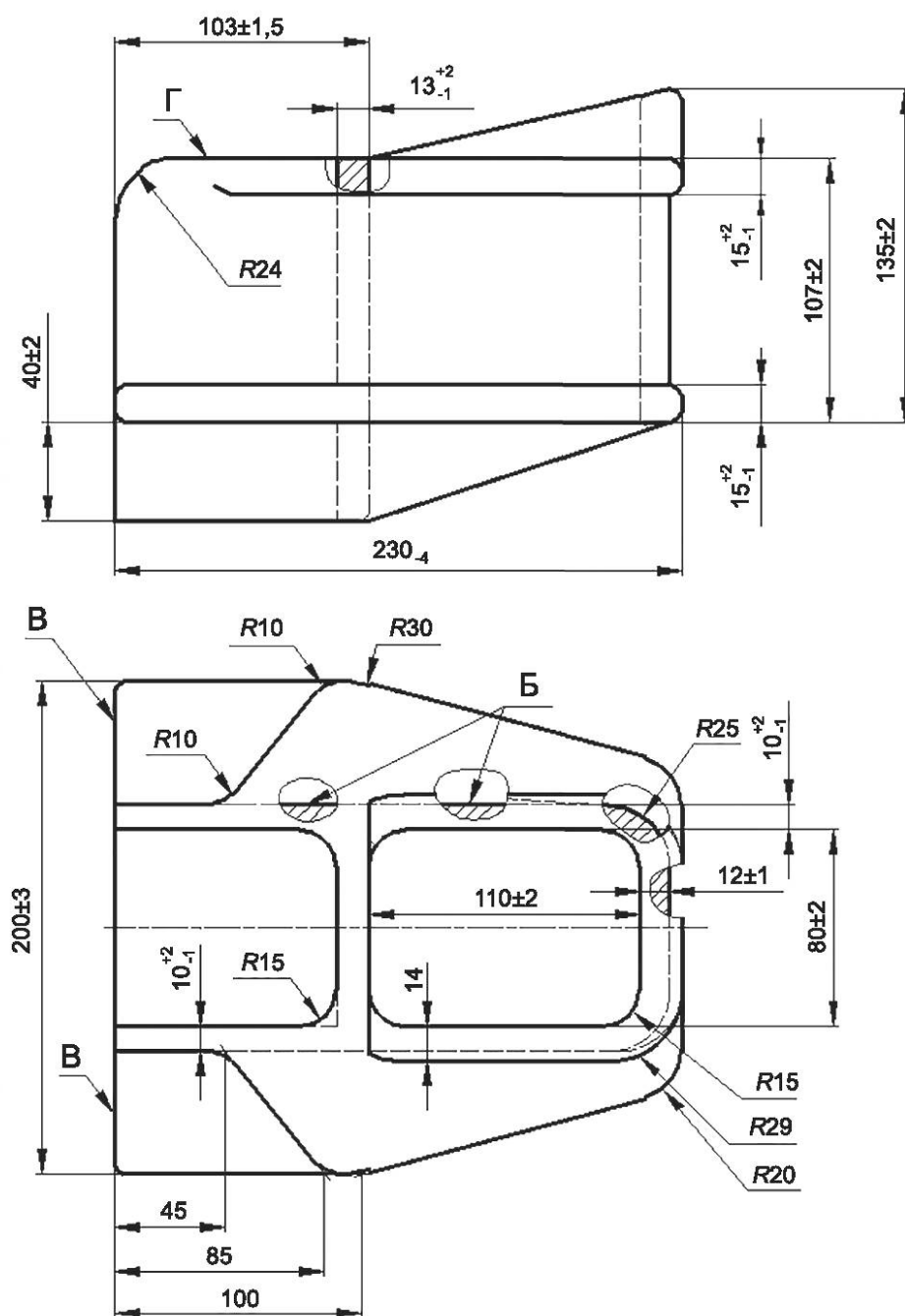
Рисунок 3 — Стоечная скоба типа III исполнения -02
