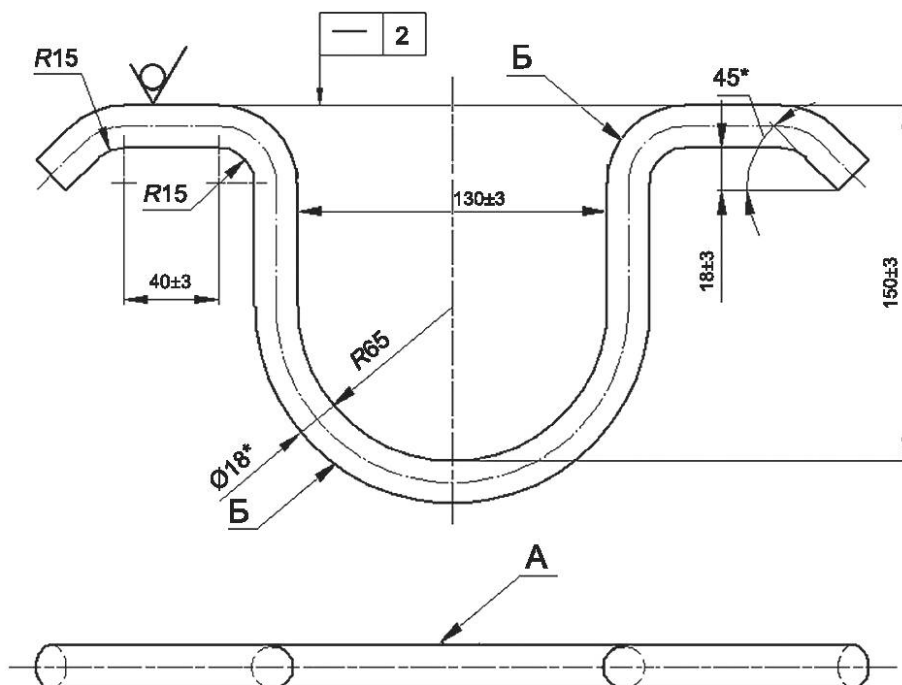
а) Исполнение -01
