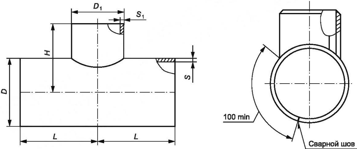
Рисунок 7 — Тройник сварной
