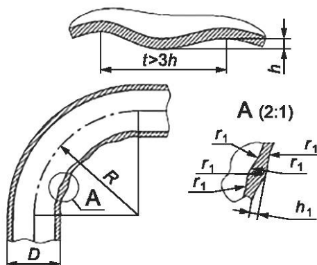
Рисунок 5 — Дефекты поверхности горячекнутых отводов
