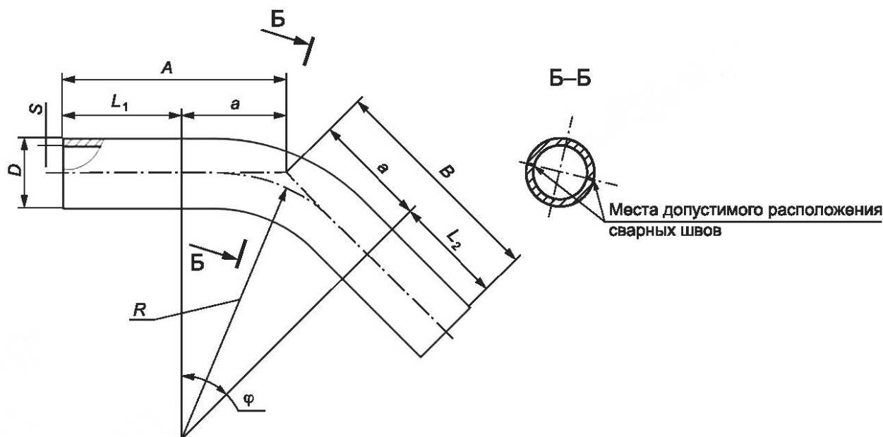
Рисунок 4 — Отвод горячегнутый
