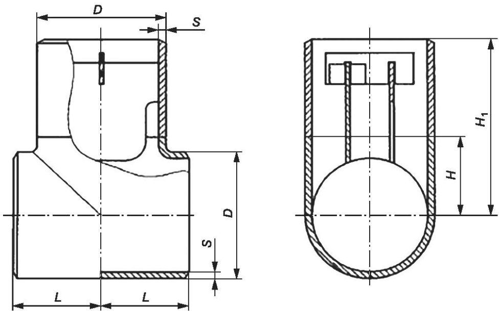
б) Размеры и конструкция равнопроходных и переходных тройников с решеткой Рисунок 8 — Размеры тройников с решетками
