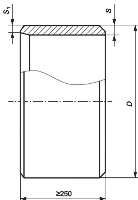
Рисунок 11 — Кольцо переходное
