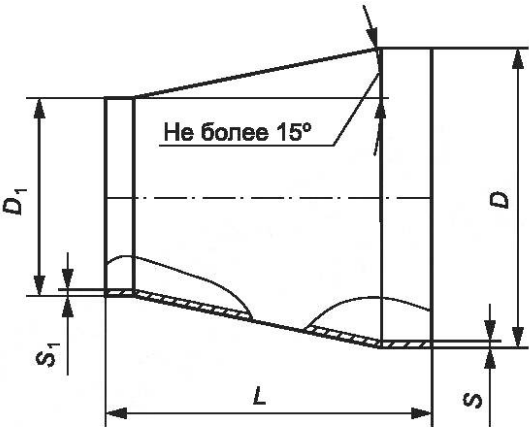
а) Переходы штамповарные
