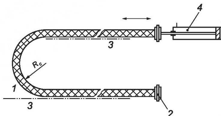
1 — испытуемый гибкий рукав; 2 — закрепленный конец рукава; 3 — опора для рукава; 4 — цилиндр для подачи сжатого воздуха (длина хода поршня 250 мм)
