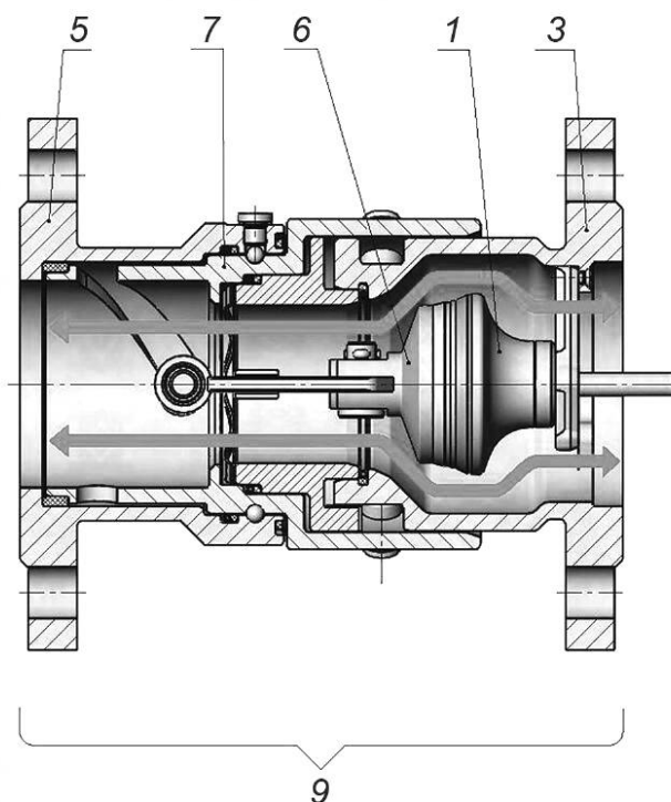
1 — внутренний клапан; 3 — корпус адаптера; 5 — корпус соединителя; 6 — поршень; 7 — ротор; 9 — сухое разъёмное соединение в сборе
