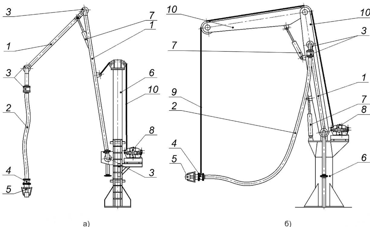
1 — трубопровод; 2 — гибкий рукав; 3 — шарнирное соединение; 4 — муфта аварийного разъединения; 5 — сухое разъёмное соединение; 6 — стойка; 7 — гидроцилиндр; 8 — механизм подъёма/опускания; 9 — трос подъёма/опускания; 10 — стрела
