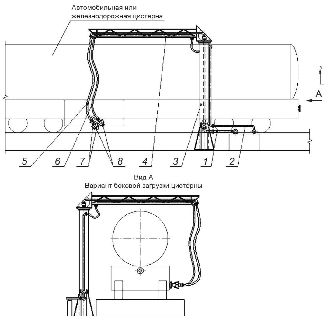
1 — трубопровод СПГ; 2 — трубопровод отпарных газов; 3 — стойка; 4 — поворотная стрела; 5 — гибкий рукав (шланг) СПГ; 6 — гибкий рукав (шланг) отпарных газов; 7 — муфта аварийного разъединения; 8 — сухое разъемное соединение
