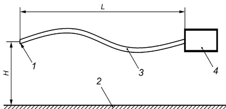
1 — точка подключения гибкого рукава (шланга); 2 — горизонтальный бетонный пол; 3 — гибкий рукав (шланг); 4 — муфта
