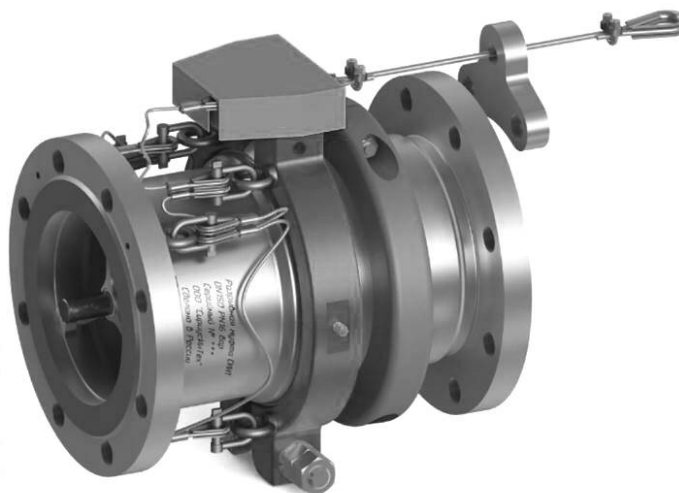
Рисунок 2 — Тросовая (пассивная/активная) муфта аварийного разъединения
