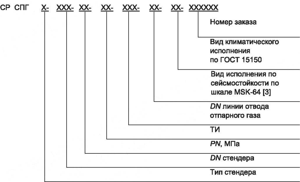
Рисунок 1 — Схема условного обозначения стэндера
