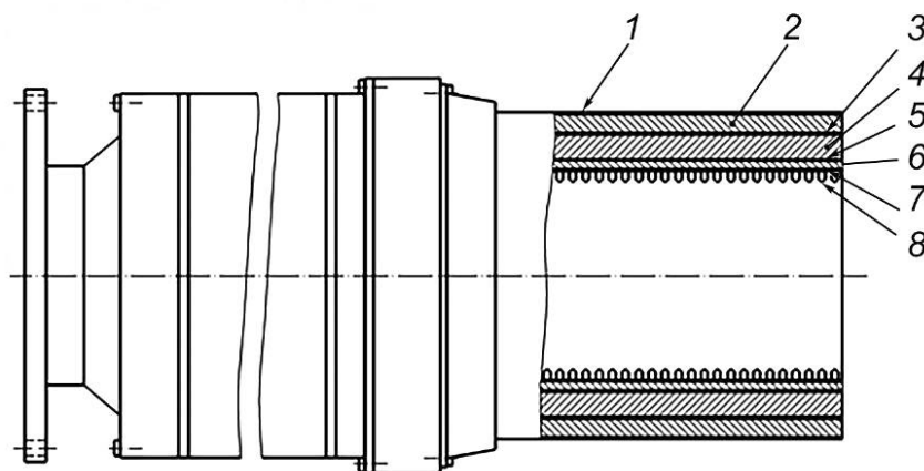
1 — герметичный слой; 2 — изоляция; 3 — герметичный слой; 4 — изоляция; 5 — поддерживающий слой; 6 — армирование; 7 — герметичный слой; 8 — внутренний гофрированный рукав
