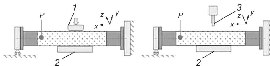
1 — сжимающая пластина; 2 — поддерживающая пластина; 3 — ударное приспособление
