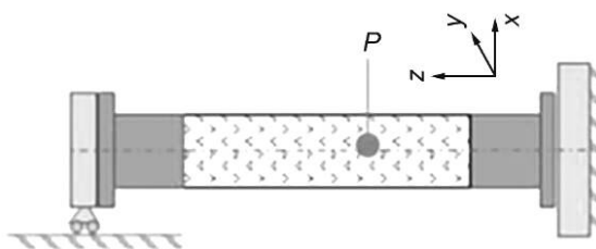
Рисунок 9 — Принцип испытаний давлением в условиях окружающей среды и низких температур
