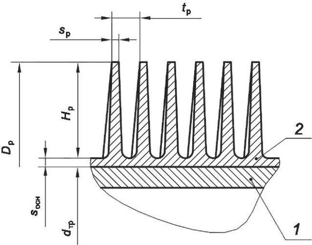
1 — несущая теплообменная труба; 2 — оребрение (ребра); d_{тр} — наружный диаметр несущей теплообменной трубы; D_p — наружный диаметр по оребрению теплообменной трубы; t_p — шаг ребер; s_p — толщина конца ребра; H_p — высота ребра (от основания до конца ребра); s_{оч} — толщина от наружной поверхности несущей трубы до основания ребра
