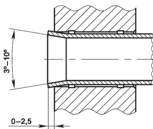
Рисунок 7 — Схема предварительной развальцовки конца теплообменной трубы
