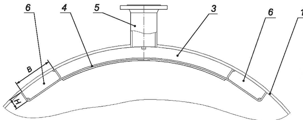
а) Вид сборника обезвоженного продукта в сечении электродегидратора
