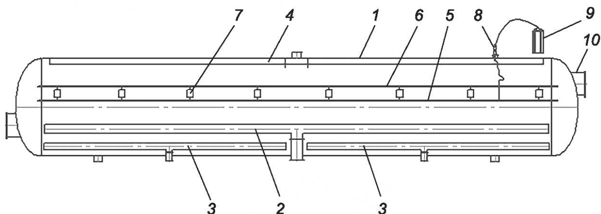
Рисунок 1 — Типовая конструкция вертикального электродегидратора
