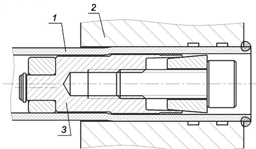
1 — теплообменная труба; 2 — трубная решетка; 3 — ПЗВ
