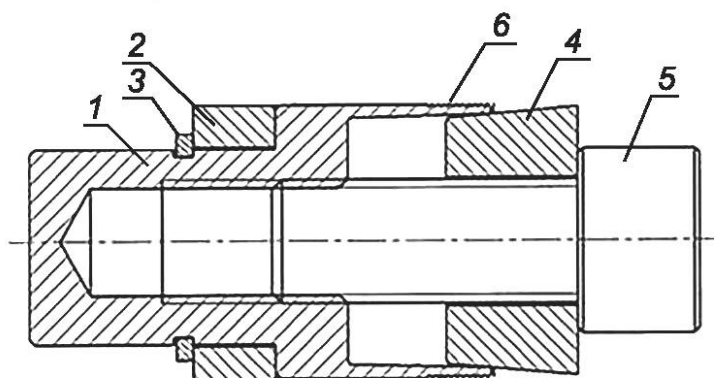
а) ПЗВ исполнения 1 для глушения теплообменной трубы
