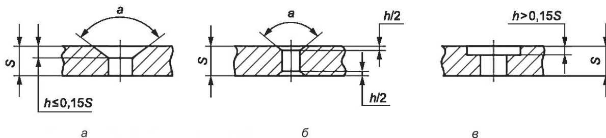
Рисунок 8 — Схема зенковки
