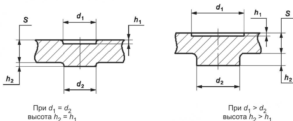
Рисунок 9 — Схема высадки
