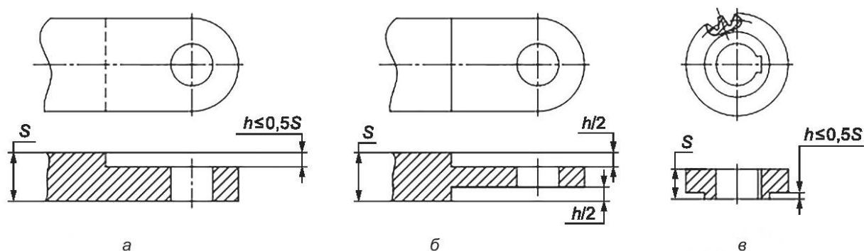
Рисунок 10 — Схема осадки
