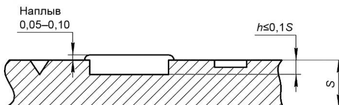
Рисунок 7 — Схема рельефной чеканки
