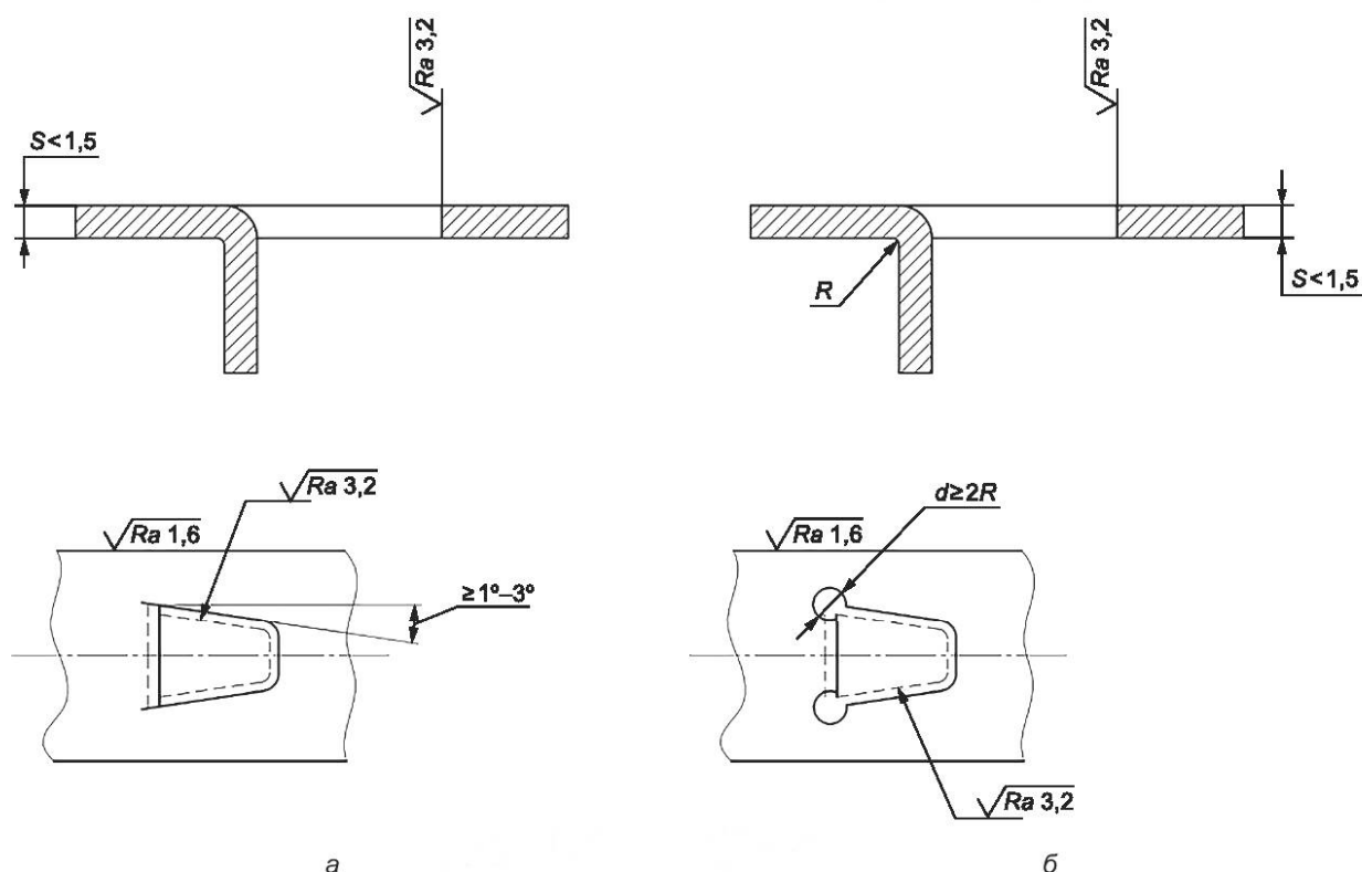
Рисунок 4 — Схема надрезки с отгибкой
