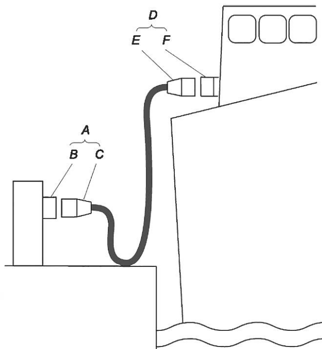
А — (береговая) вилка и розетка; В — (береговая) розетка; С — (береговая) вилка; D — судовой соединитель; E — судовой разъем; F — вводной порт питания
