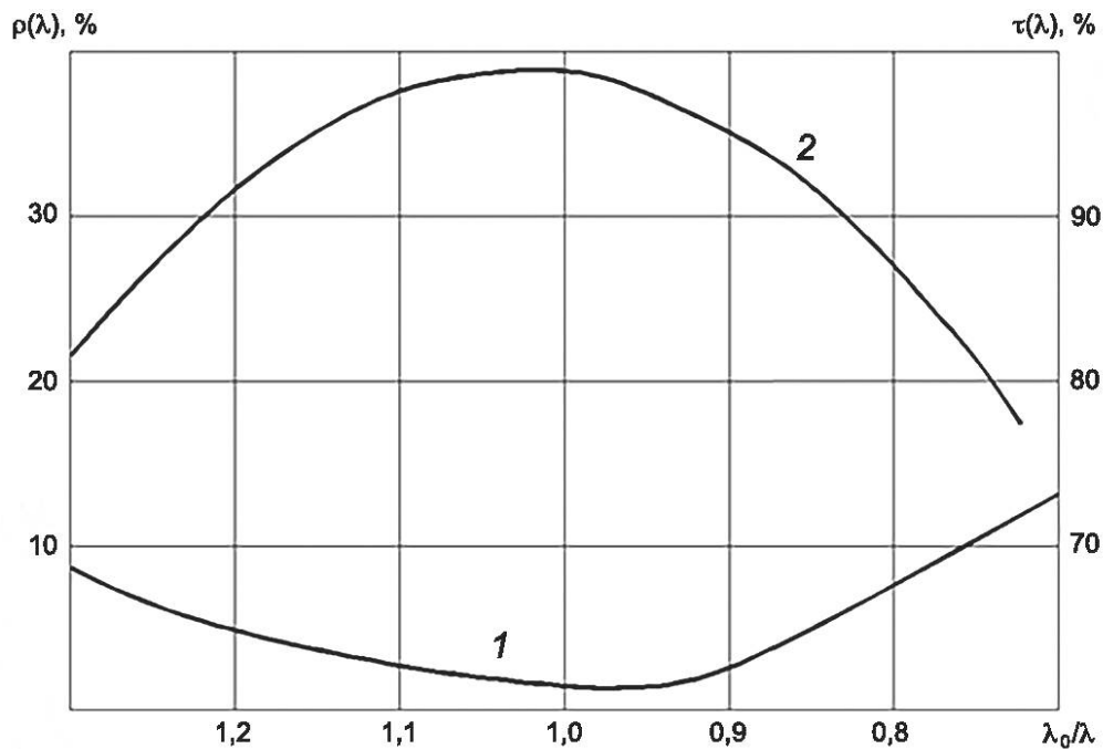
Рисунок Б.3 — Спектральные кривые коэффициентов отражения (кривая 1) и пропускания (кривая 2) просветляющего покрытия 29IIt на деталях из германия
