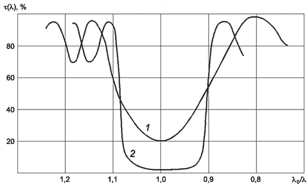
Рисунок Б.4 — Спектральные кривые коэффициентов отражения (кривая 1) и пропускания (кривая 2) просветляющего покрытия (39I:37I) \times m:39I , где m = 2 (кривая 1) и m = 8 (кривая 2) на деталях из фтористого кальция
