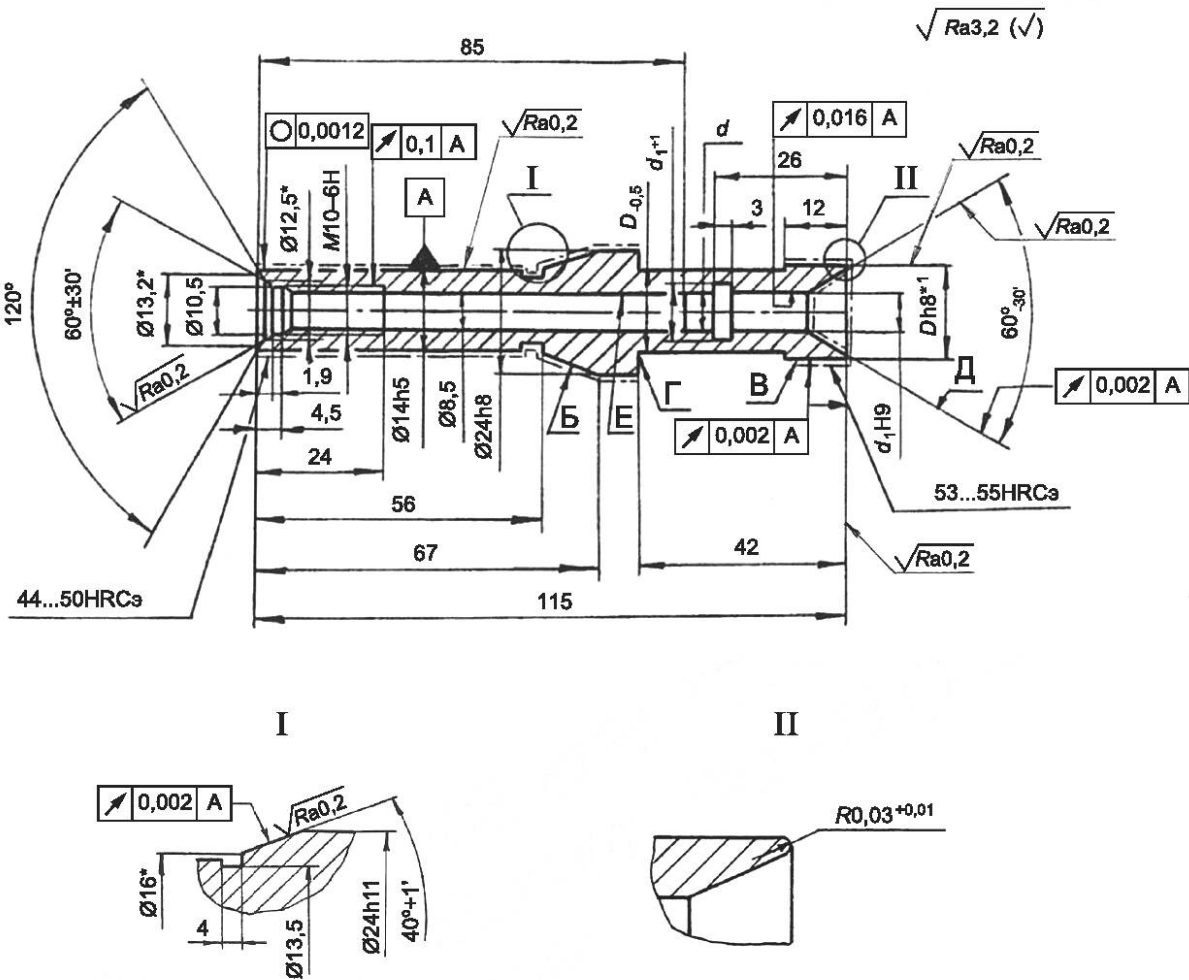
a — для D_{\text{л}} от 10 до 24 мм включительно
