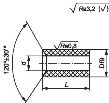
Рисунок 7 — Конструкция и размеры втулок
