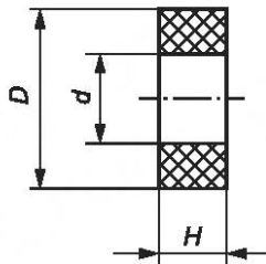
Рисунок 8 — Размеры вкладышей
