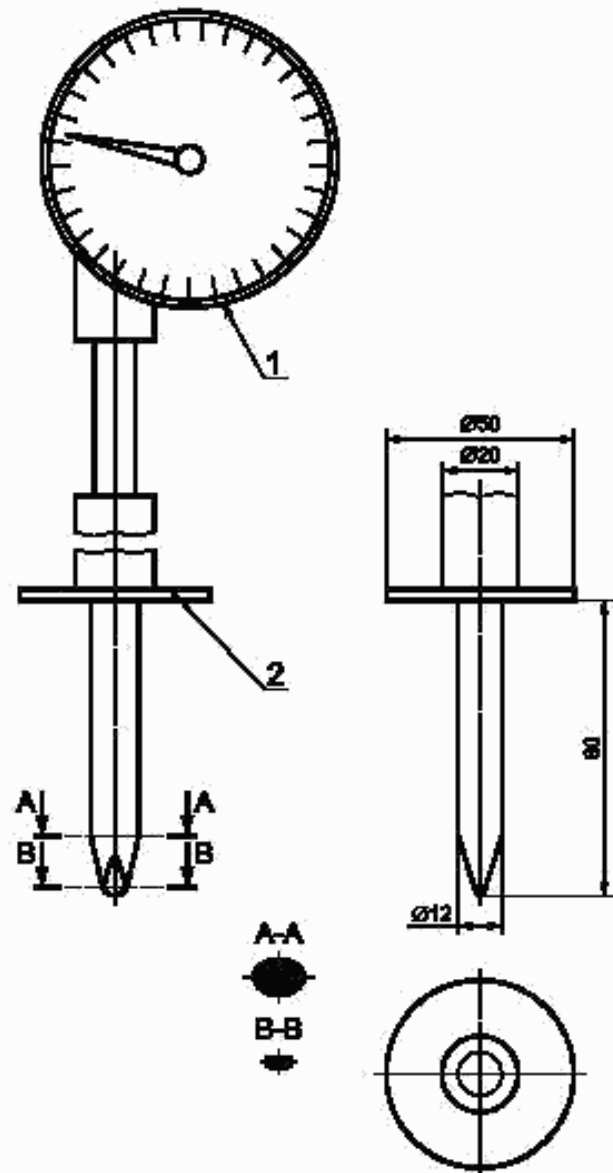
Рисунок А.2 — Пример стандартного нешарнирного (прямого) испытательного пальца
