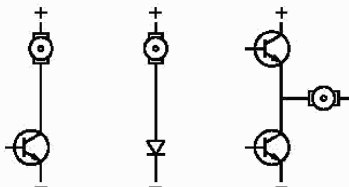
а) Выходные цепи основного контура
