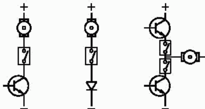
с) Испытательные переключатели, подключенные к разомкнутой цепи
