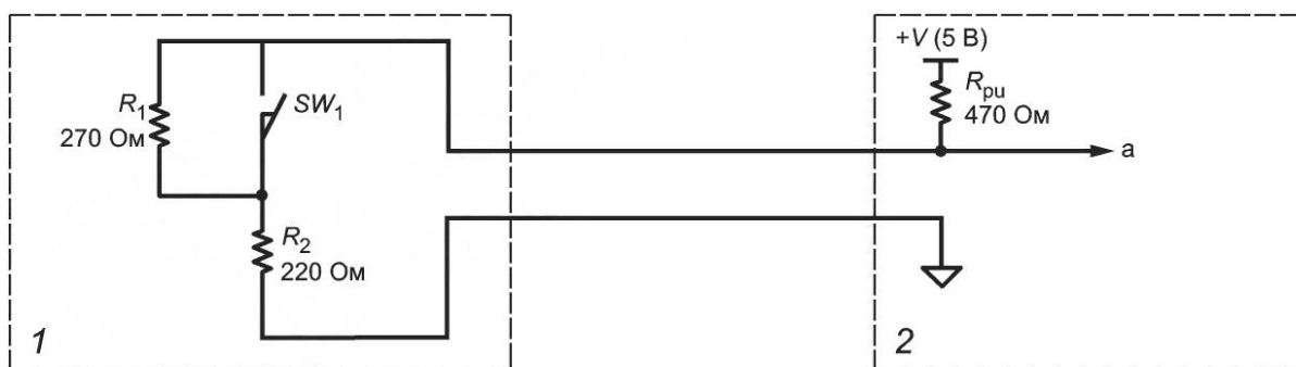
Рисунок С.1 — Предлагаемая схема интерфейса выключателя
