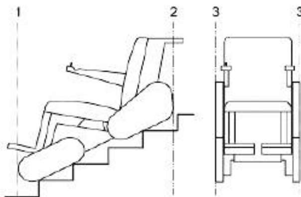
1 — передняя вертикальная плоскость (3.19); 2 — задняя вертикальная плоскость (3.35); 3 — боковая вертикальная плоскость (3.40)
