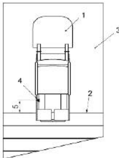
1 — ограничитель пространства для сопровождающего; 2 — окровка ступени под номером 8; 3 — верхняя лестничная площадка; 4 — базовая метка; 5 — расстояние между окровкой ступени под номером 8 и базовой меткой
