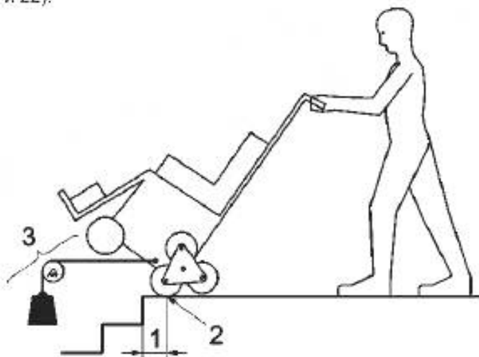
1 — начальное расстояние (100 \pm 10) мм; 2 — самая передняя точка контакта; 3 — устройство ускорения (пример)
