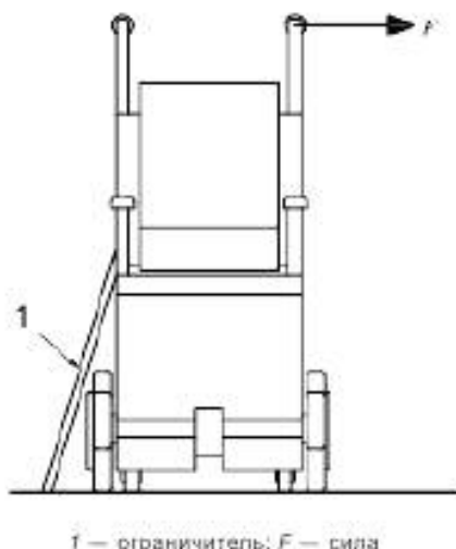
Рисунок 27 — Приложение направленной вбок силы к ручкам устройства для преодоления лестниц
