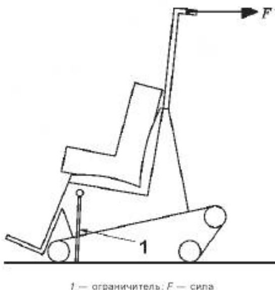
Рисунок 25 — Приложение направленной назад силы к ручкам самоустанавливающегося устройства для преодоления лестниц
