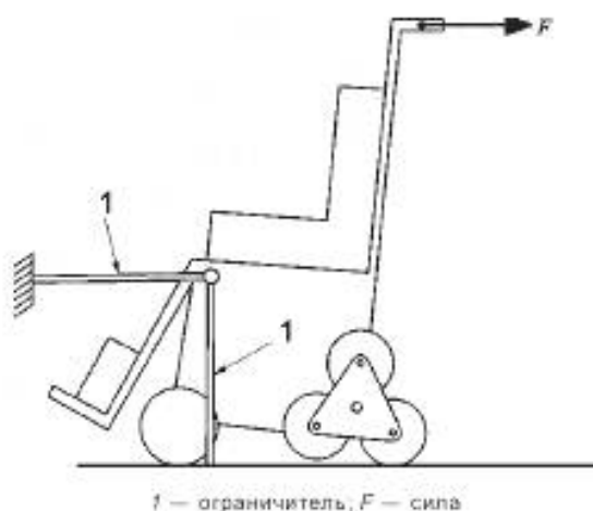
Рисунок 26 — Приложение направленной назад силы к ручкам устройства для преодоления лестниц, стабилизируемого вручную
