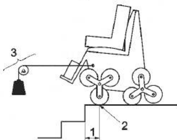
1 — начальное расстояние (100 \pm 10) мм; 2 — самая передняя точка контакта; 3 — устройство ускорения (пример)
