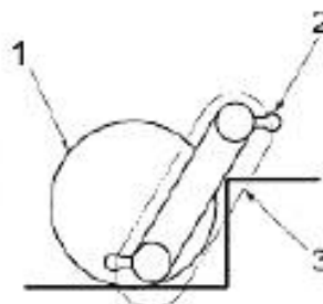
1 — нижний исполнительный механизм (колесо); 2 — верхний исполнительный механизм (палец); 3 — траектория самой нижней точки пальца относительно механизма преодоления
