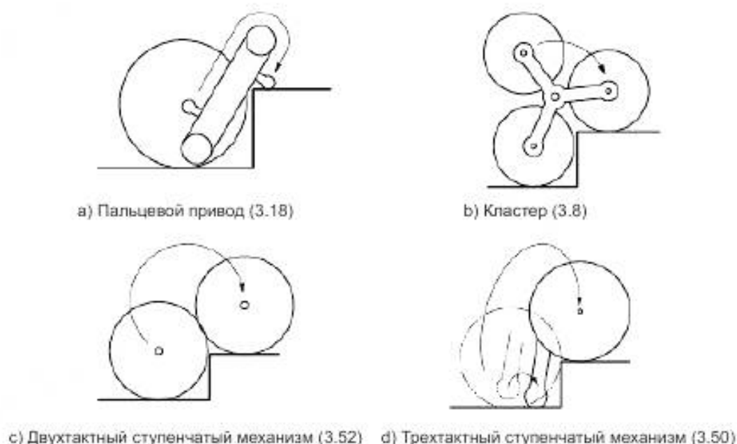
Рисунок 8 — Примеры ступенчатых механизмов преодоления
