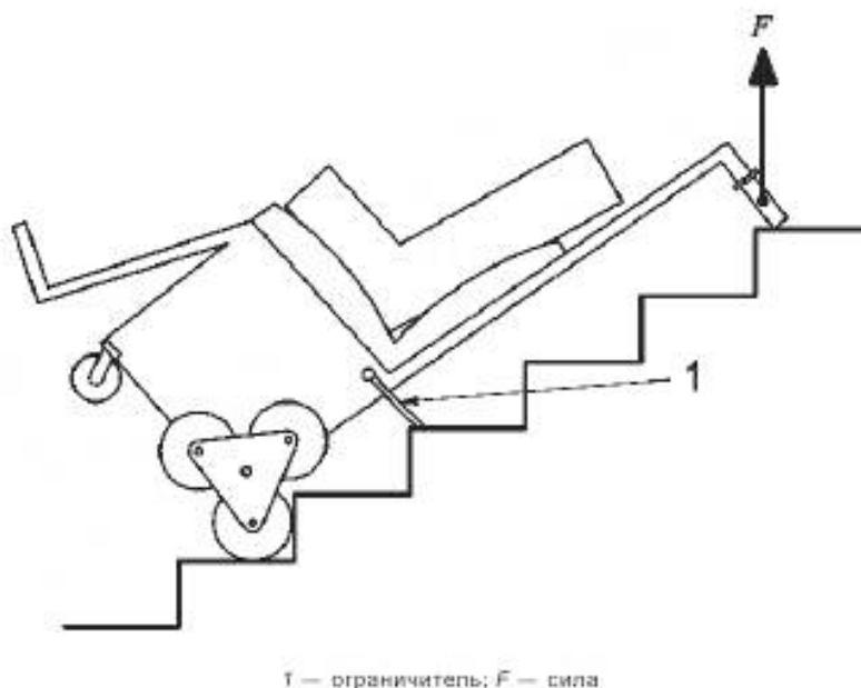
Рисунок 24 — Приложение нагрузки, направленной вверх, к ручкам устройства для преодоления лестниц, стабилизируемого вручную
