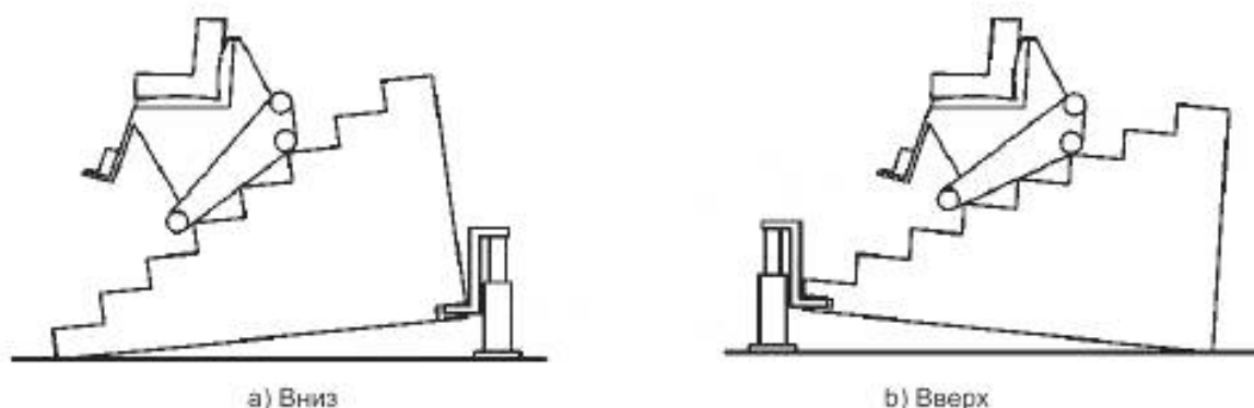
Рисунок 13 — Пример подъемного механизма с наклоненной испытательной лестницей
