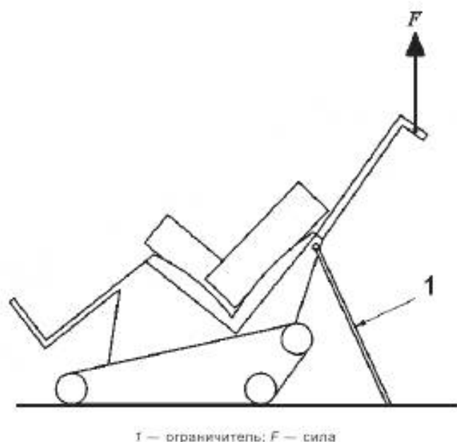
Рисунок 23 — Приложение направленной вверх силы к ручкам самоустанавливающего устройства для преодоления лестниц
