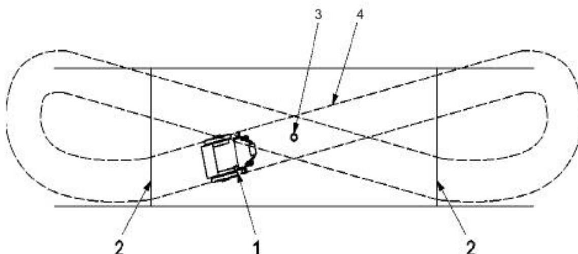
1 — кресло-коляска; 2 — маркер; 3 — центральный маркер; 4 — пример пути кресла-коляски
