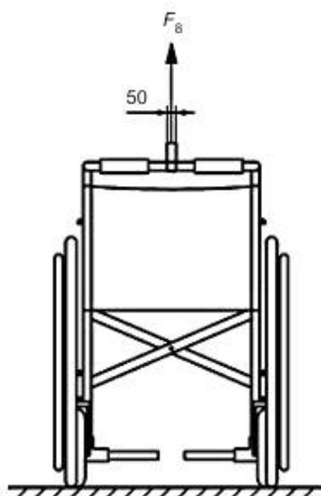
b) сила, прикладываемая к рукоятке в виде перекладины снизу вверх
