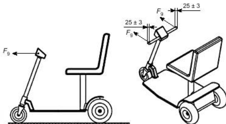
Рисунок 19 — Силы, прикладываемые к рукояткам управления скутером
