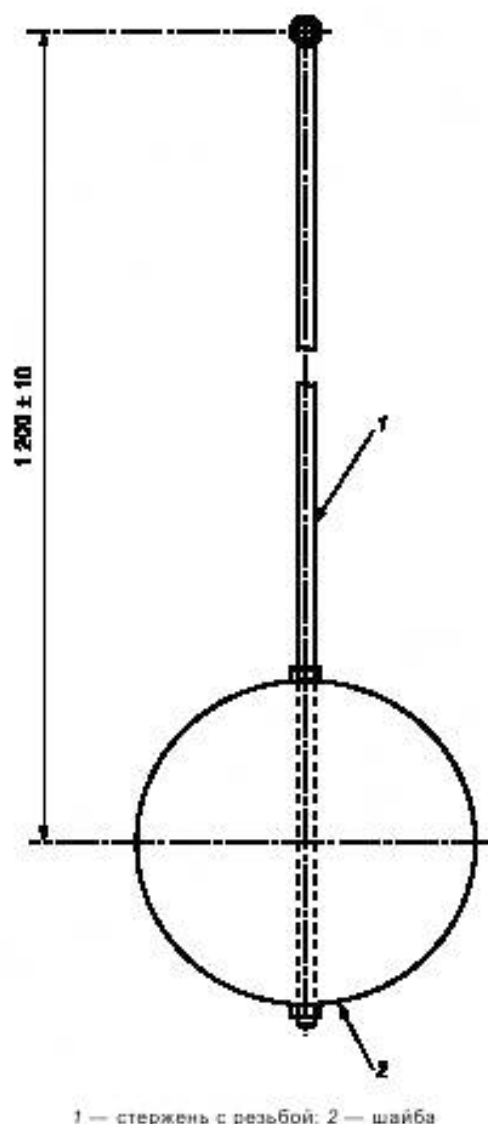
Рисунок 4 — Альтернативный маятник для испытания спинки кресла
