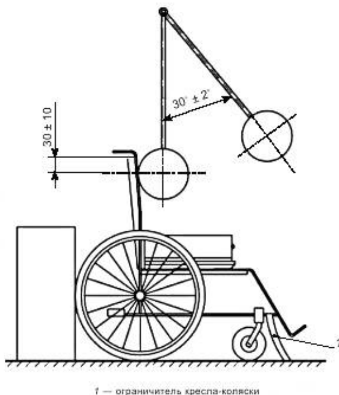
Рисунок 24 — Испытание на ударную прочность спинки кресла
