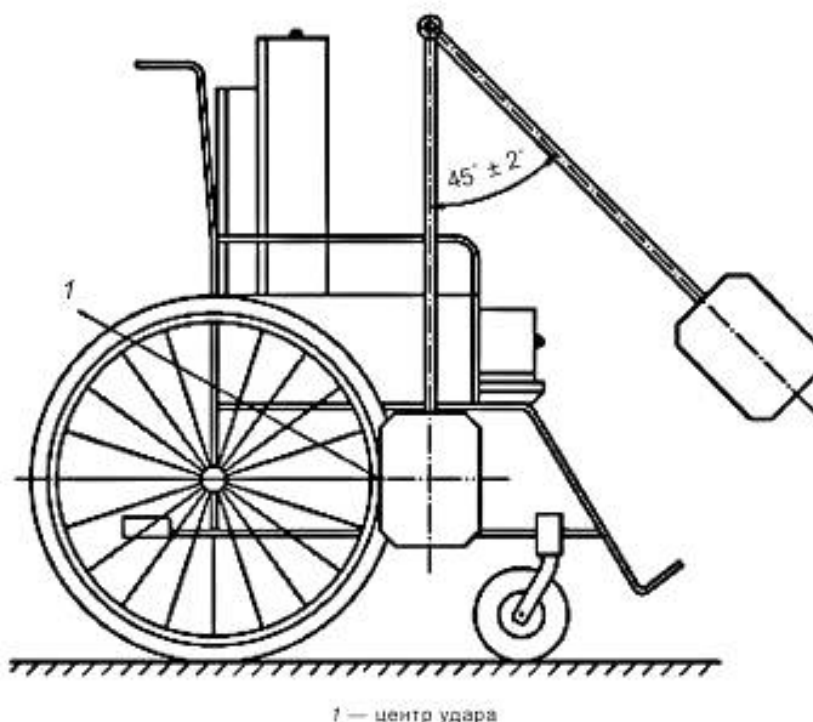
Рисунок 25 — Испытание обода ручного привода на ударную прочность
