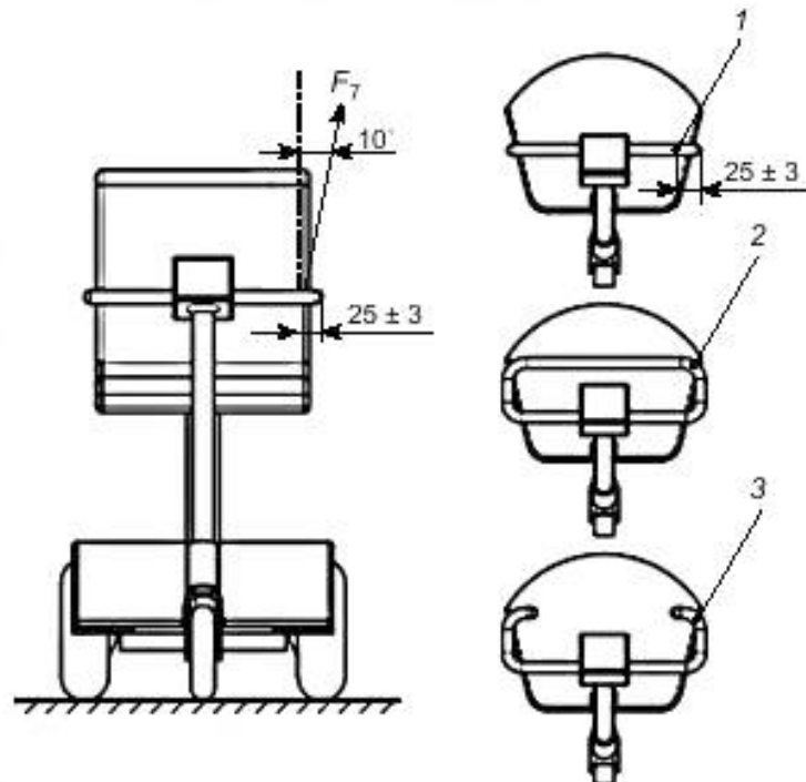
Рисунок 21 — Силы, прикладываемые к рукоятке управления скутером сверху вниз
