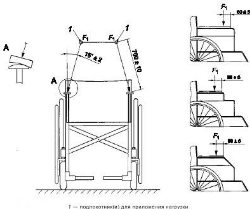
Рисунок 10 — Силы, направленные сверху вниз, и подлокотники
