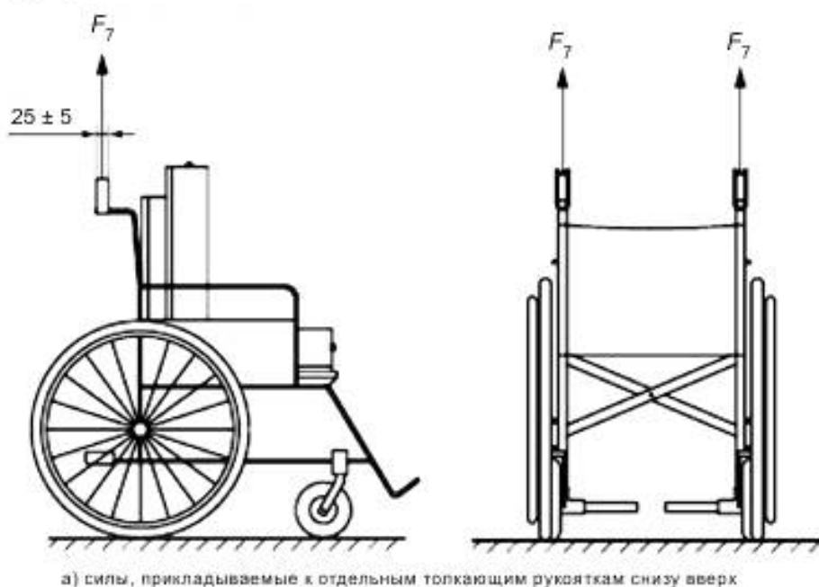
Рисунок 18 — Силы, прикладываемые к толкающим рукояткам снизу вверх
