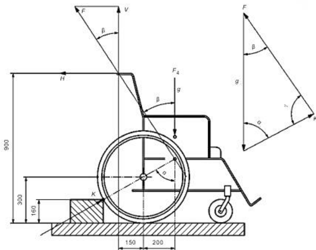
Рисунок А.2 — Нагрузки кресла-коляски на бордюрном камне
