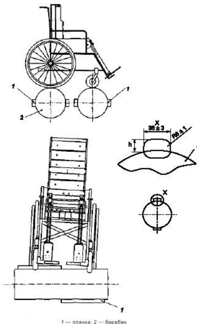
Рисунок 6 — Мультибарабанный испытательный стенд
