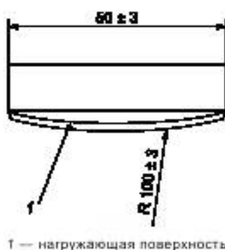
Рисунок 2 — Выпуклая нагружающая пластина
