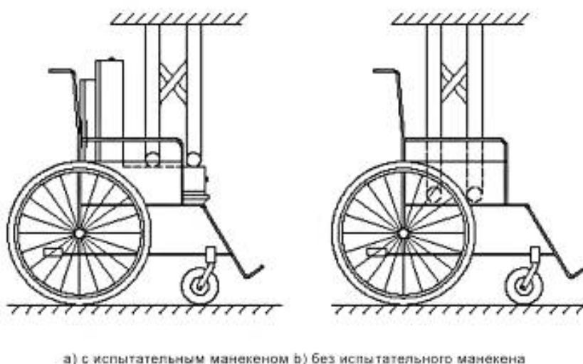
Рисунок 7 — Метод предохранения кресла-коляски от опрокидывания
