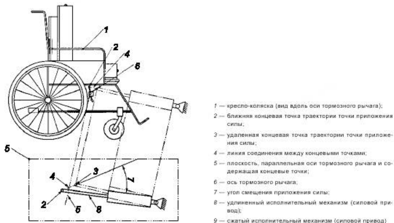
Рисунок 9 — Иллюстративная настройка системы повторяющегося действия тормоза
