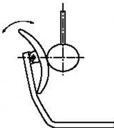
Рисунок 23 — Разворачивающаяся спинка кресла
