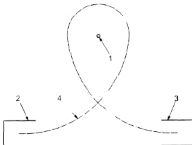
1 — отметка М; 2 — прямоугольник А; 3 — прямоугольник В; 4 — траектория движения кресла-коляски
