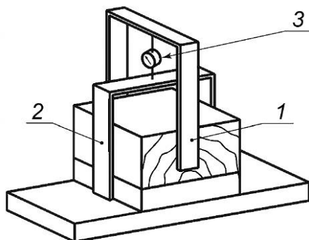
1 — скоба, зажимающая шашку; 2 — скоба, нажимающая на доску; 3 — прибор, измеряющий усилие, направленное на отрыв шашки от доски
