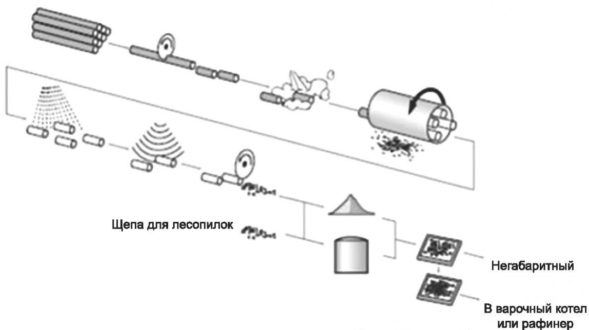
Рисунок 2 — Схема производства щепы
