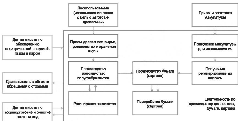
Рисунок 1 — Блок-схема целлюлозно-бумажного производства
