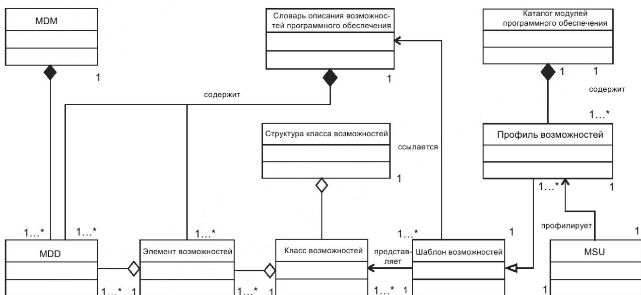
Рисунок 5 — Взаимосвязь между каталогом модулей программного обеспечения и другими компонентами
