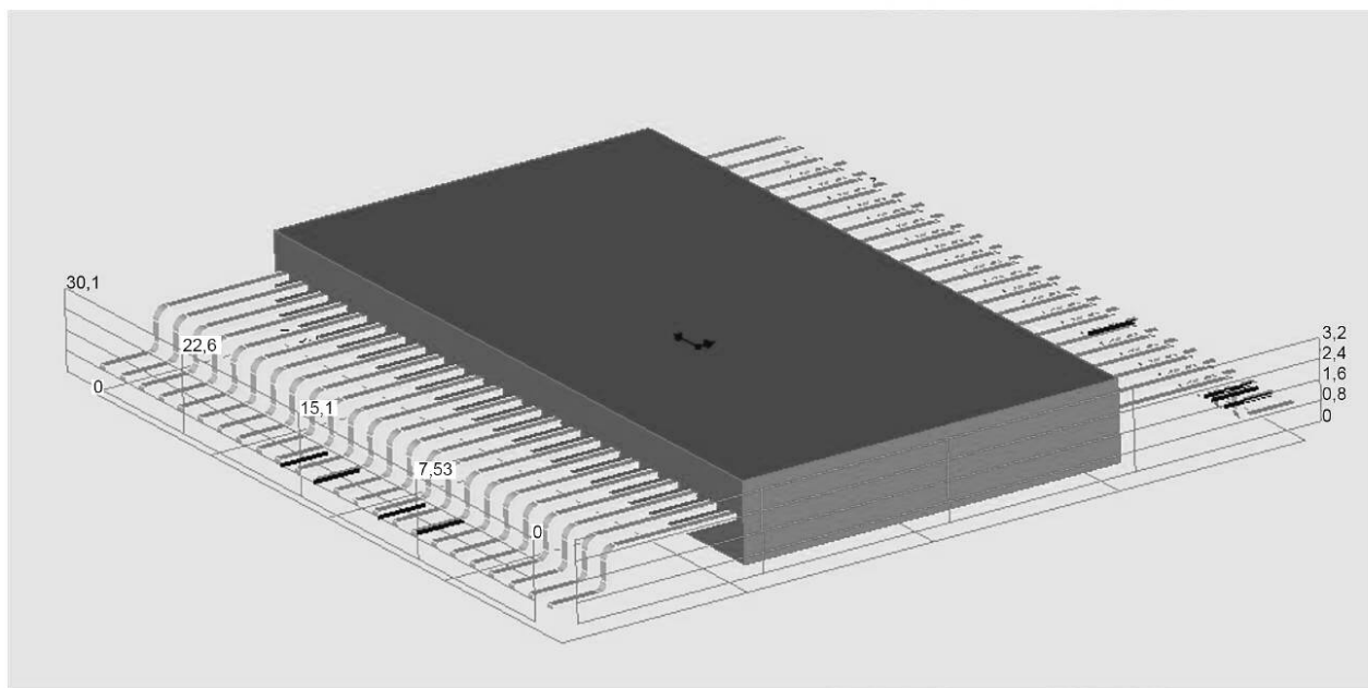
Рисунок А.1 — Конструкция ЭКБ, импортированная из САД-системы в подсистему АСОНИКА-М-3D
