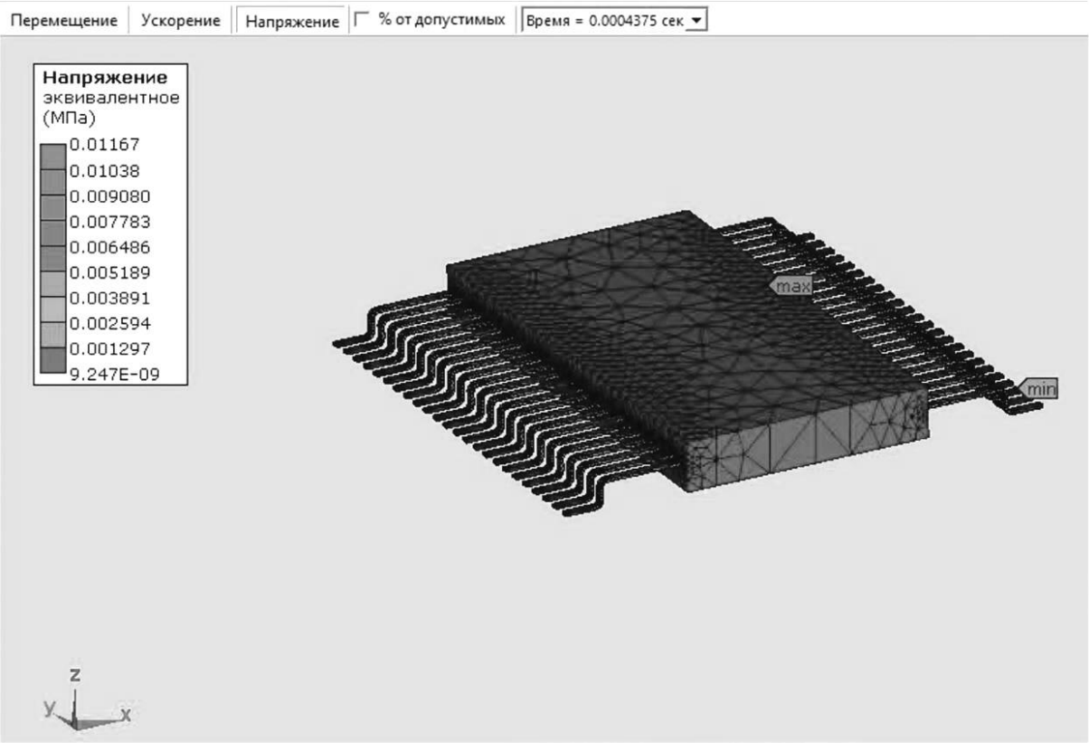
Рисунок А.8 — Эквивалентные механические напряжения во всех точках конструкции ЭКБ при воздействии одиночного механического удара в заданный момент времени
