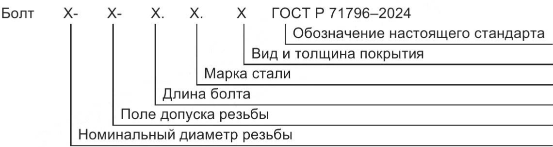
Рисунок 6 — Схема формирования условного обозначения болтов
