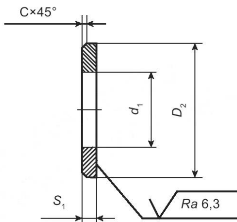
Рисунок 9 — Конструкция шайбы
