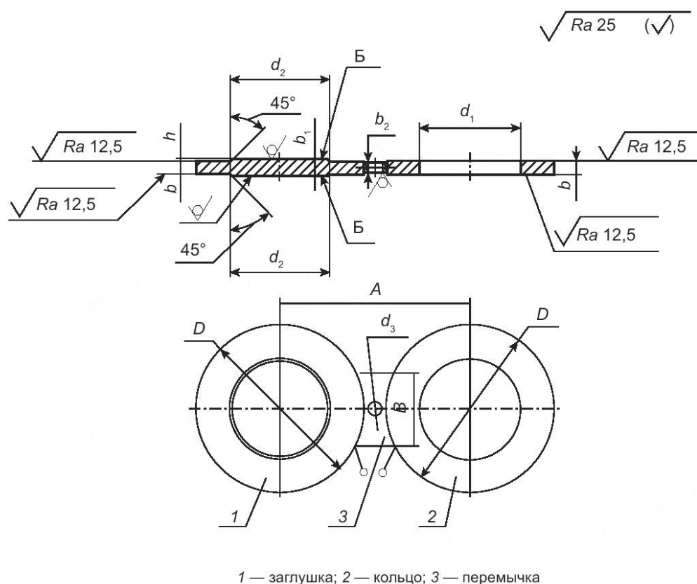
Рисунок 1 — Конструкция поворотной заглушки типа 1
