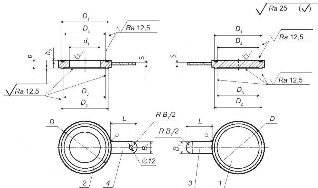
1 — заглушка; 2 — кольцо; 3 — хвостовик без отверстия; 4 — хвостовик с отверстием
