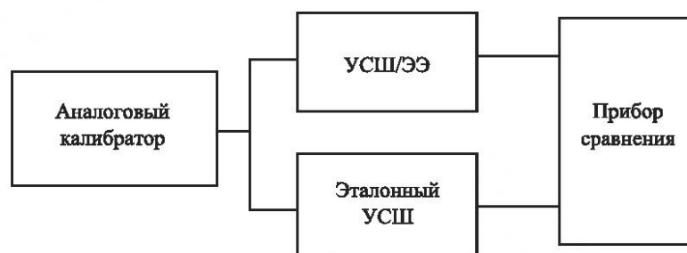
Рисунок А.2 — Схема испытаний точности УСШ/ЭЭ с применением аналогового калибратора без внешней синхронизации
