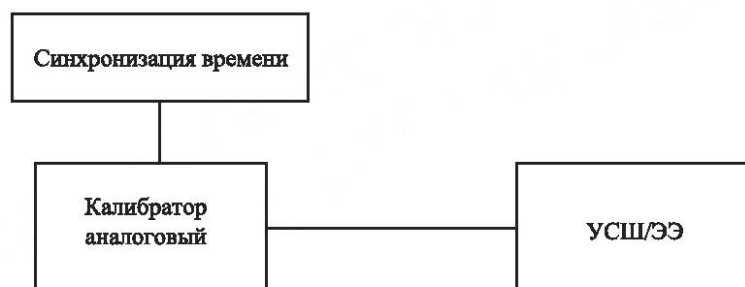
Рисунок А.1 — Схема испытаний точности УСШ/ЭЭ с применением аналогового калибратора с возможностью внешней синхронизации по 1PPS сигналу или протоколу PTP
