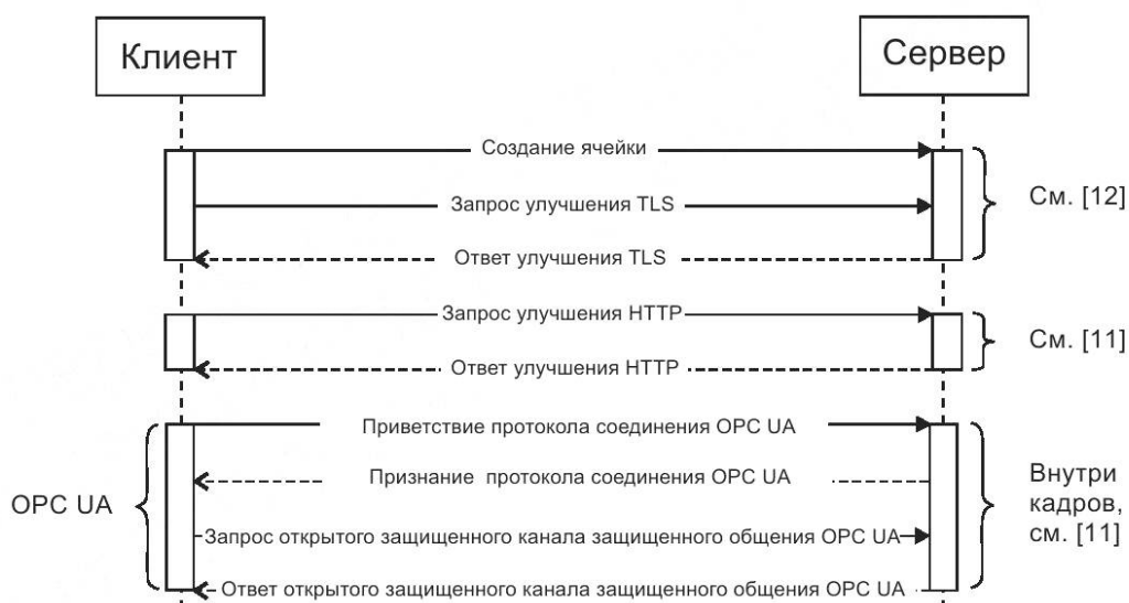
Рисунок 17 — Настройка связи через WebSocket
