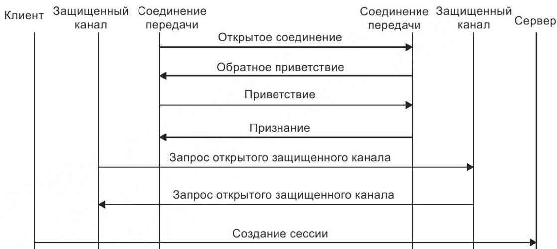
Рисунок 14 — Иницированное сервером соединение по протоколу соединения OPC UA
