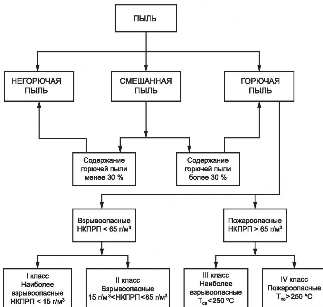
Рисунок Г.1 — Классификация пыли
