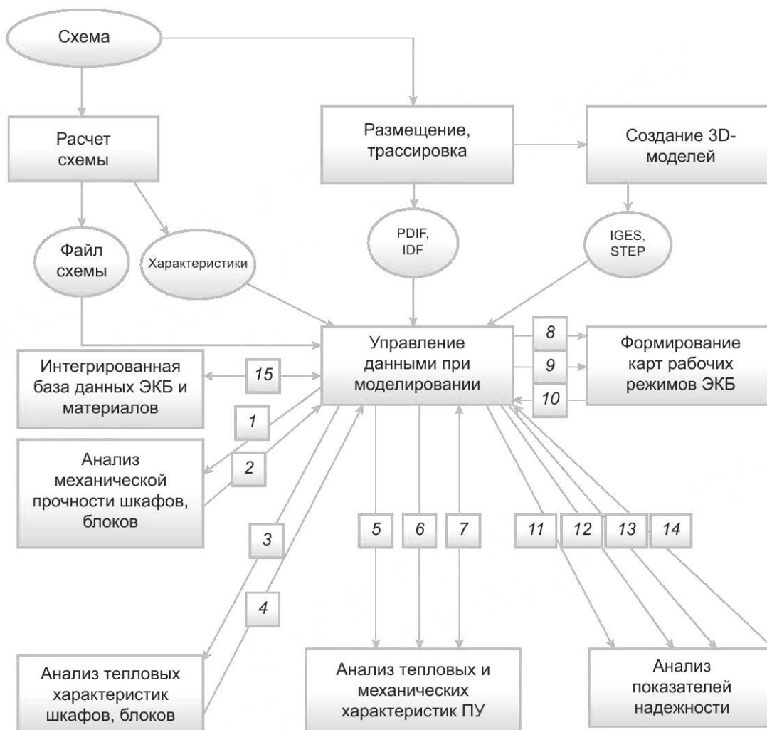
Рисунок 1 —Технология создания KPP ЭКБ на основе математического моделирования и виртуализации испытаний ЭКБ и ЭА на ВВФ при проектировании
