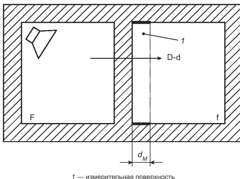
1 — измерительная поверхность
