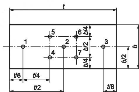
Рисунок И.1 — Схема измерения остаточных толщин листа
