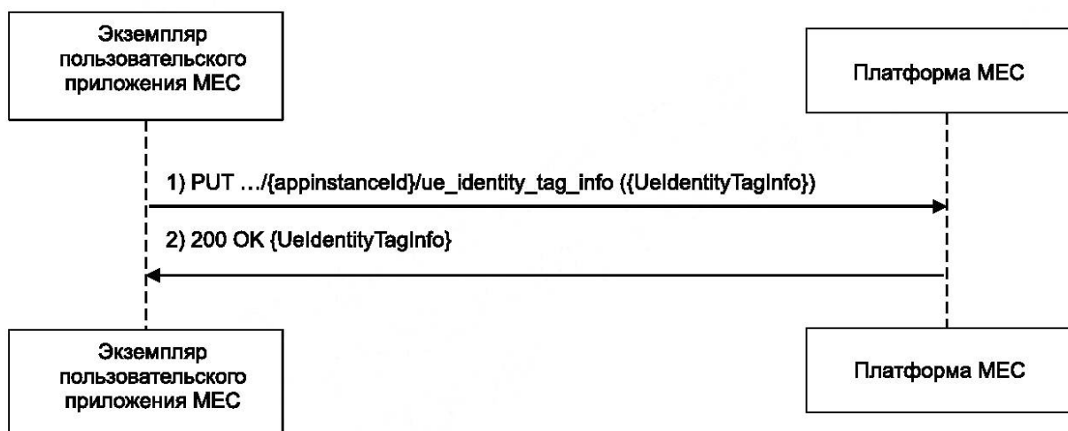
Рисунок 2 — Процесс регистрация тега идентификации UE
