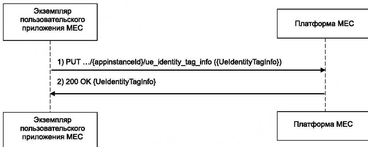
Рисунок 3 — Процесс отмены регистрации тега идентификации UE
