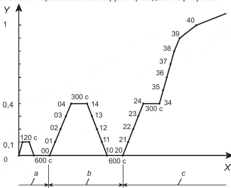
а) Уровень горизонтальной нагрузки в зависимости от времени
