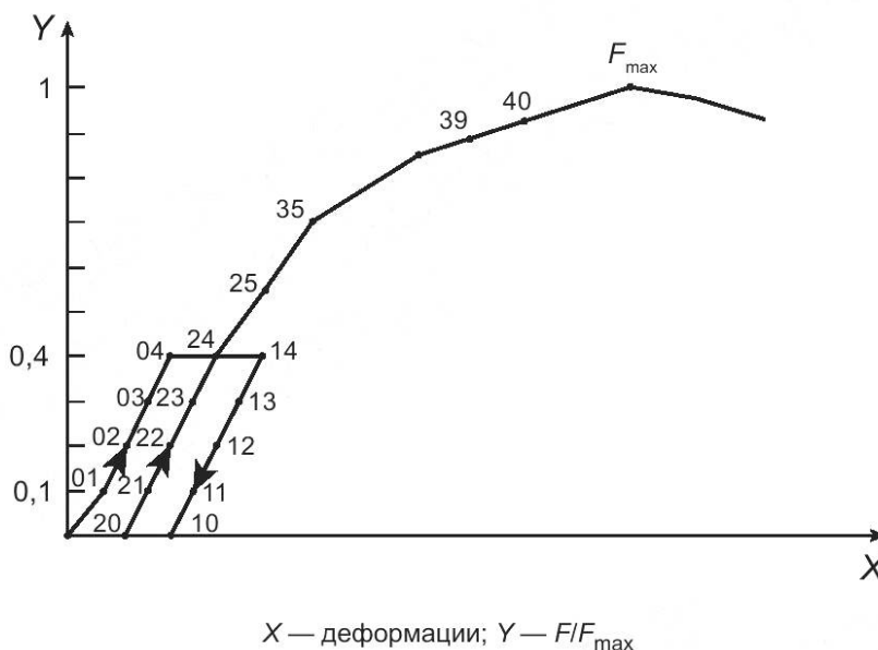
б) Зависимость деформации от горизонтальной нагрузки
