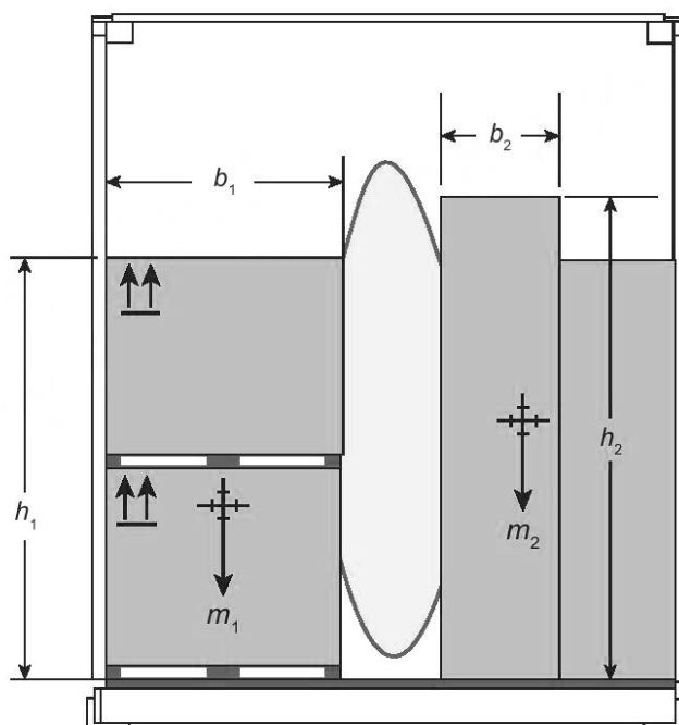
Рисунок 2 — Грузовые единицы разной высоты
