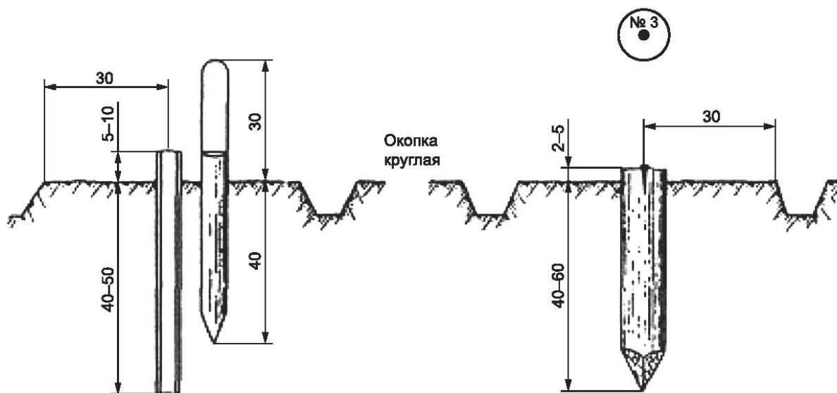
Рисунок 1 — Примеры закрепления временных пунктов СГС
