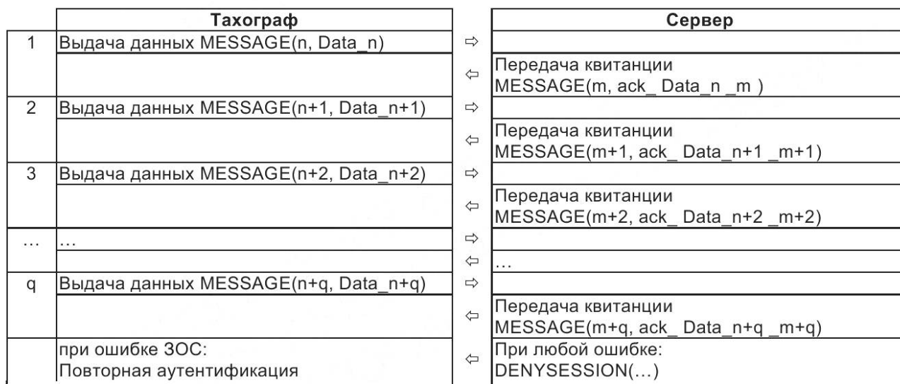
Рисунок 2 — Схема обмена сообщениями тахографа и сервера
