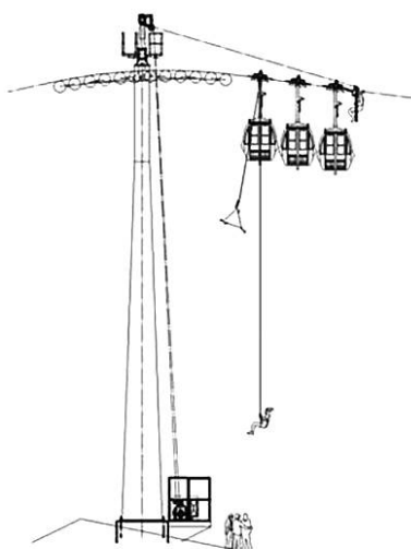
Рисунок 2 — Схема возврата подвижного состава путем перемещения его по несущему канату до линейной опоры лебедкой и эвакуации пассажиров на землю персоналом и спасателями с использованием альпинистского оборудования
