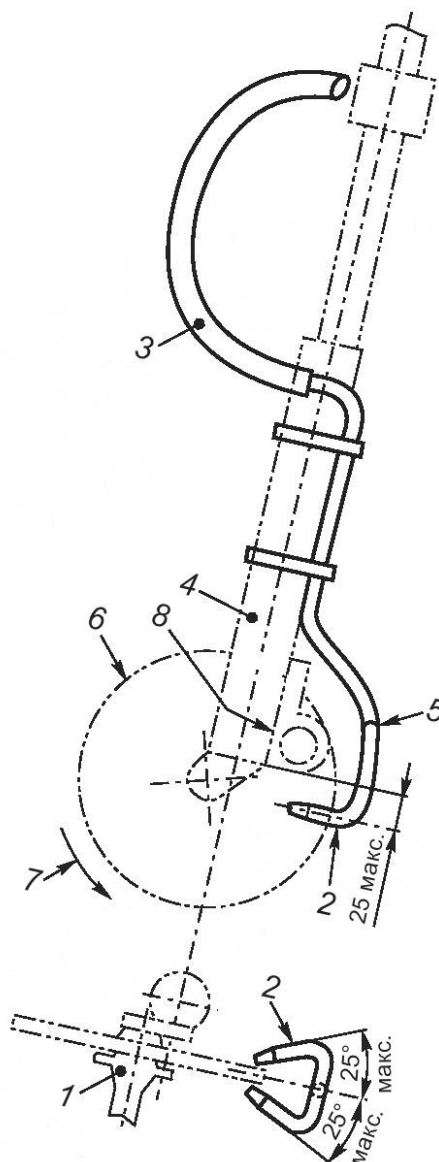
1 — передняя втулка; 2 — распылители воды; 3 — гибкая трубка; 4 — перо передней вилки; 5 — Y-образное соединение; 6 — диск тормоза; 7 — направление вращения колеса; 8 — скоба дискового тормоза
