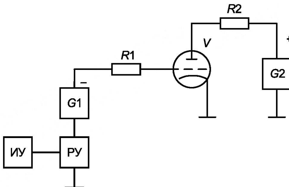
G1 — источник напряжения смещения; R1 — защитный резистор; R2 — зарядный резистор; G2 — источник питания анода; РУ — регистрирующее устройство; ИУ — индикаторное устройство
