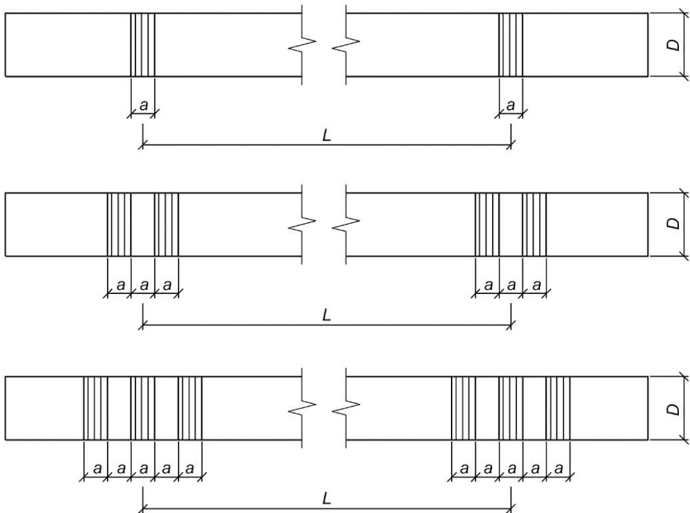
Рисунок 1 — Предупреждающие кольца
