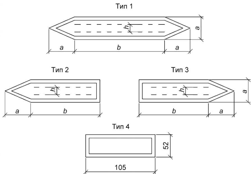
Рисунок 3 — Маркировочные щитки
