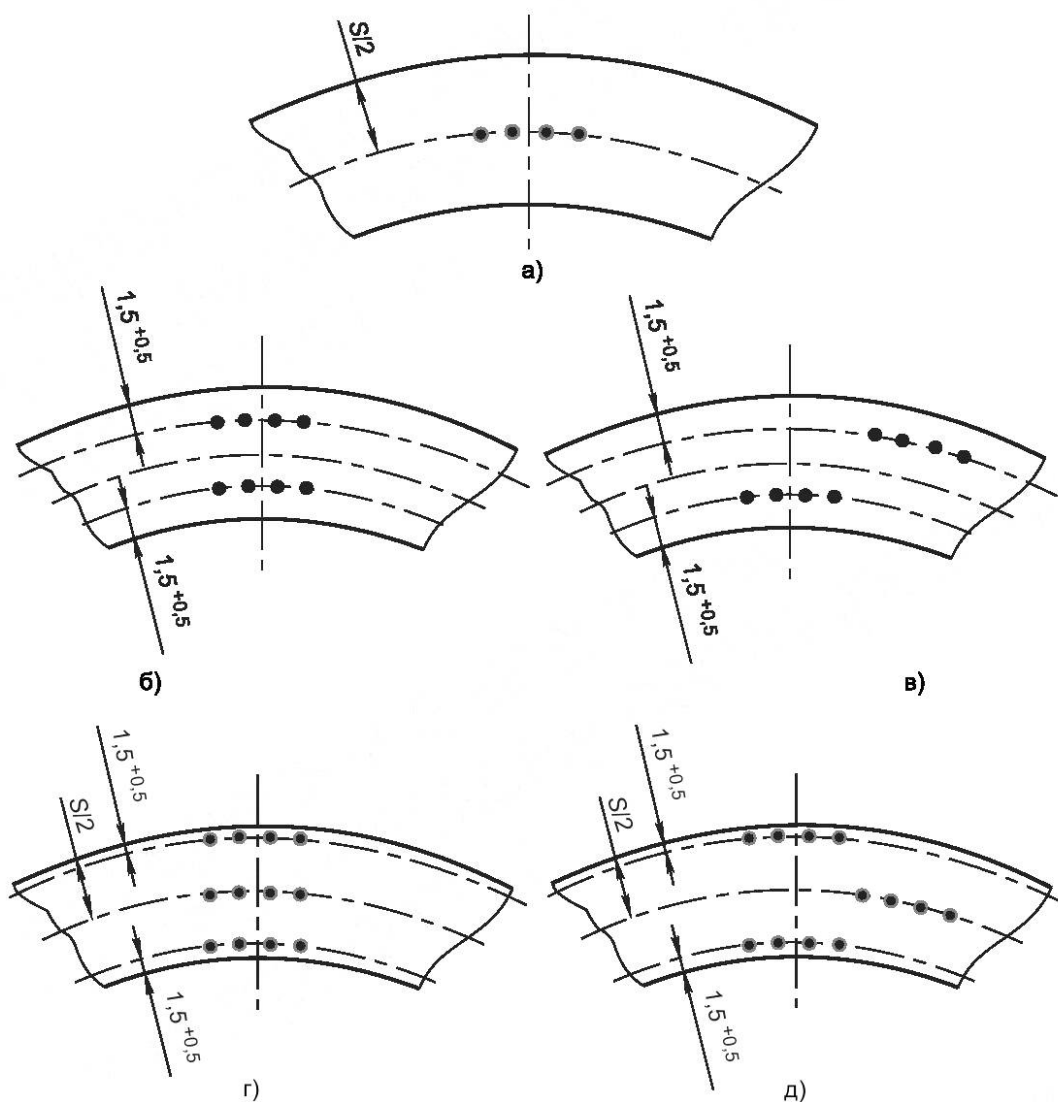
Рисунок 2 — Схема расположения отпечатка при контроле твердости
