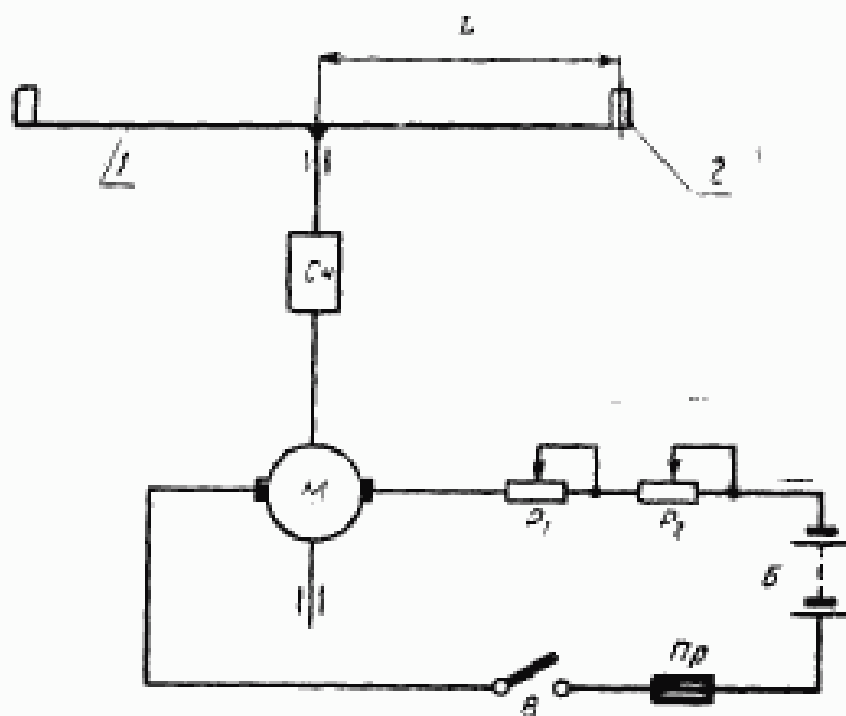
1—крестовина; 2—стойки для крепления проверяемых анемометров; Сч—счетчик числа оборотов крестовины; М—двигатель; R 1 , R 2 —резисторы; Б—аккумуляторная батарея; В—выключатель; ПР—предохранитель.
