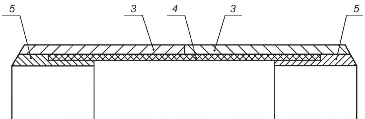
б) Образец с наконечником из трубной заготовки
